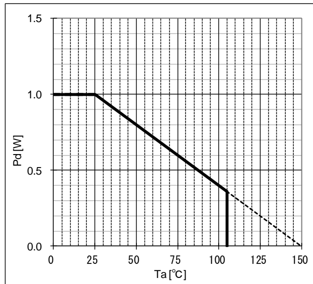
Figure 15. 熱軽減特性
