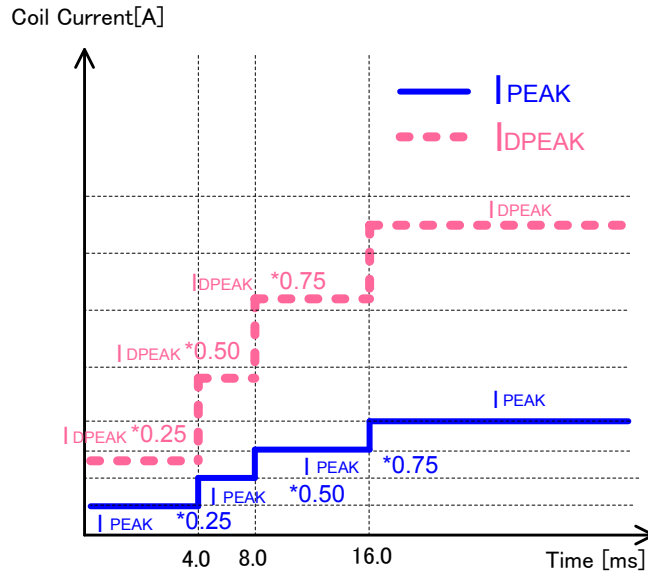
Figure 13. ソフトスタート動作
