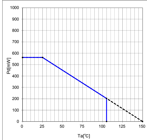
Figure 15. 熱軽減特性
