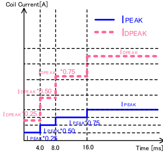
Figure 13 ソフトスタート動作
