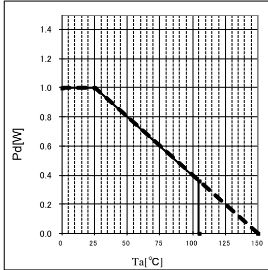
Figure 14. 熱軽減特性
