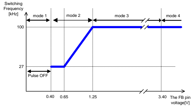
Figure 5B. スイッチング周波数 vs FB 端子電圧 (BM2P101E-Z)
