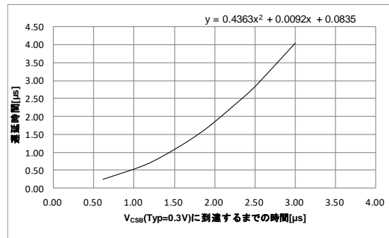
Figure 6B. 遅延時間 vs V_{CSB} (Typ=0.3 V) に到達するまでの時間(BM2P101E-Z)
