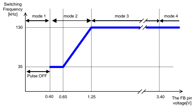
Figure 5C. スイッチング周波数 vs FB 端子電圧 (BM2P131E-Z)
