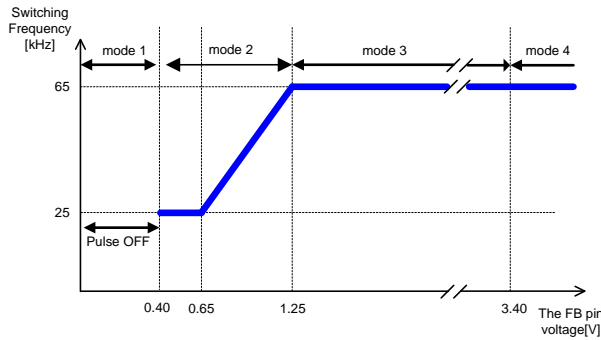
Figure 5A. スイッチング周波数 vs FB 端子電圧 (BM2P061E-Z)
