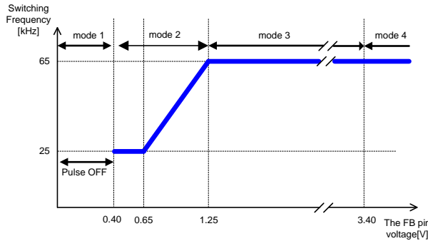
Figure 5A. スイッチング周波数 vs FB 端子電圧 (BM2P064E-Z)
