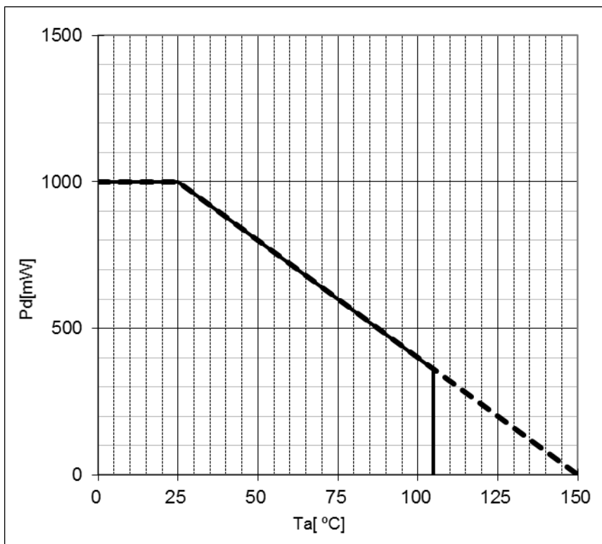
Figure 13. 熱軽減特性
