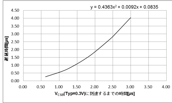
Figure 6B. 遅延時間 vs V_{CSB} (Typ=0.3 V) に到達するまでの時間(BM2P104E-Z)
