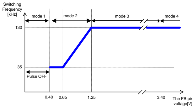
Figure 5C. スイッチング周波数 vs FB 端子電圧 (BM2P134E-Z)
