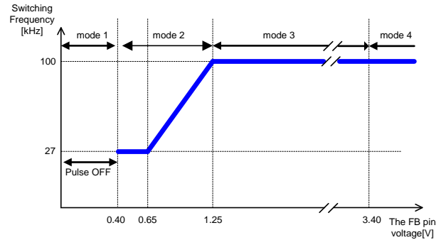
Figure 5B. スイッチング周波数 vs FB 端子電圧 (BM2P104E-Z)
