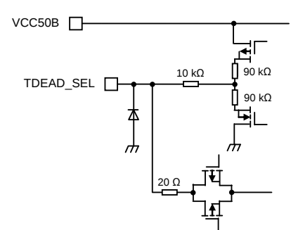
9) TDEAD_SEL pin
