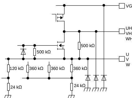
13) CP pin
