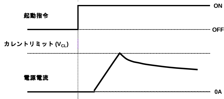
Figure 6. ソフトスタート時のコイル電流波形のタイミングチャート
