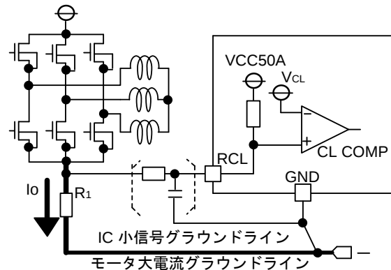
Figure 5. 小信号と大電流グラウンドライン分離
