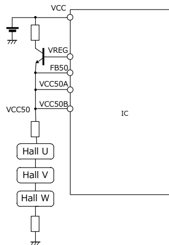
Figure 9. 外付け NPN トランジスタ使用基準電圧回路
