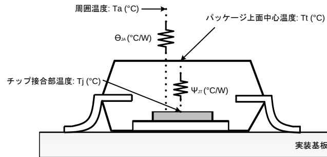
Figure 10. 表面実装パッケージの熱抵抗モデル
