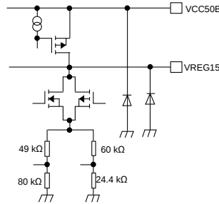
2) VREG15 pin
