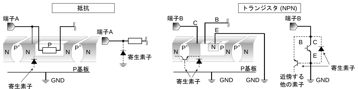
Figure 11. IC 構造例
