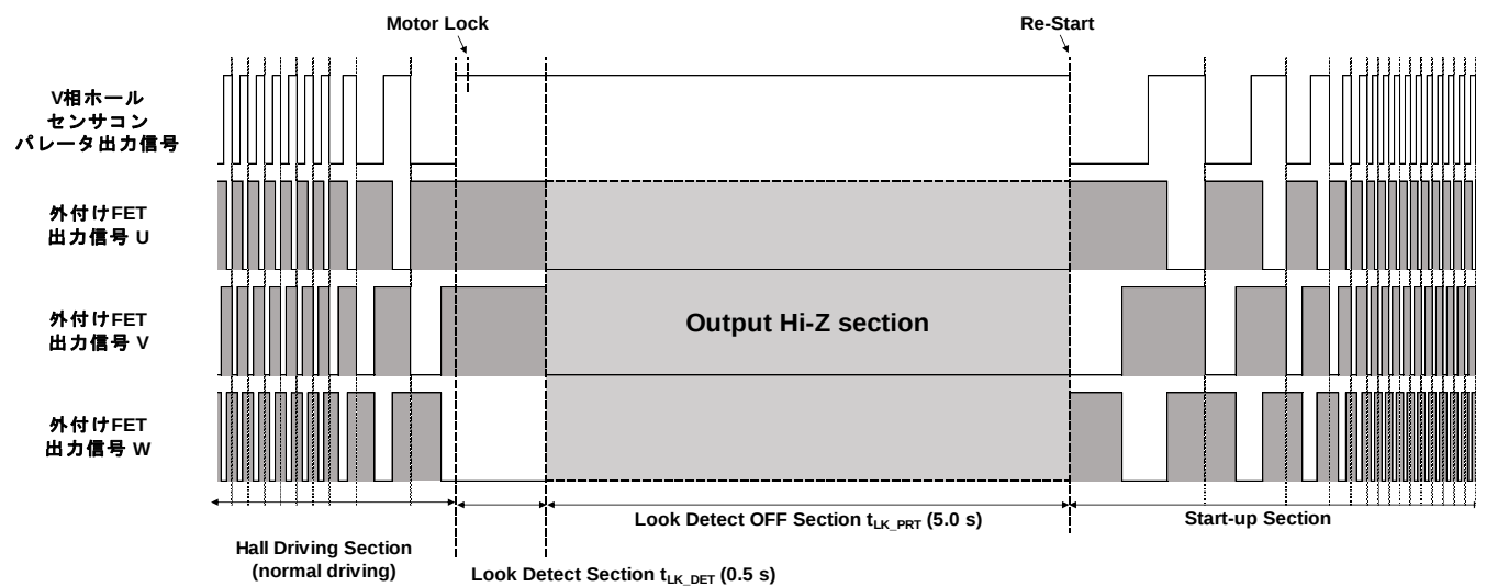
Figure 3. ロック保護時のタイミングチャート
