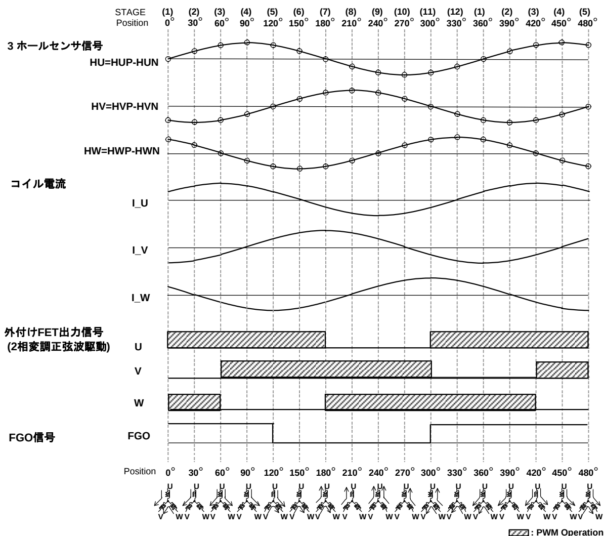
Figure 1. 正弦波駆動タイミングチャート (FR=High)
