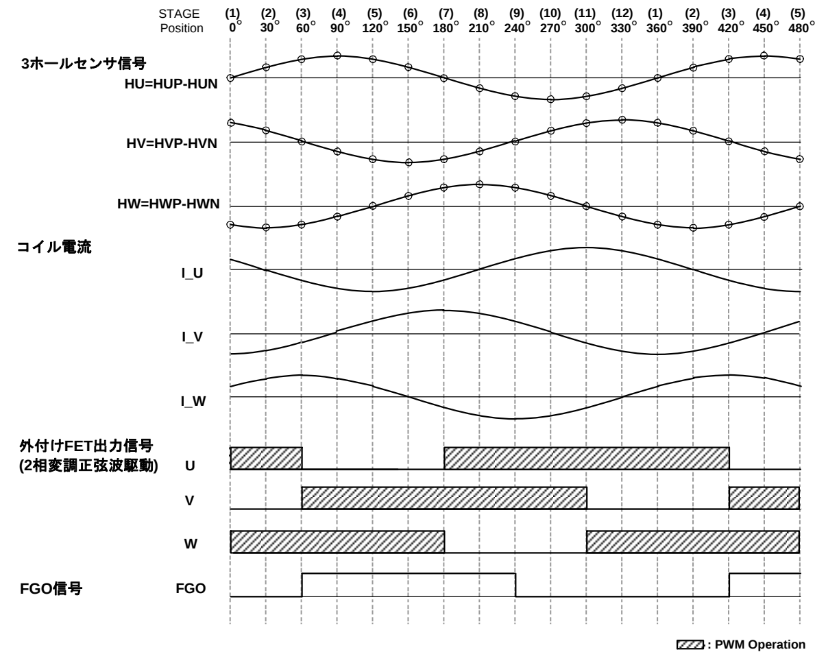
Figure 2. 正弦波駆動タイミングチャート(FR=Low)
