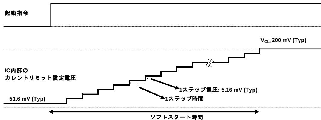
Figure 7. ソフトスタート時のカレントリミット設定電圧のタイミングチャート
