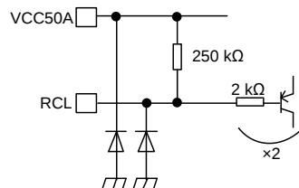
14) RCL pin
