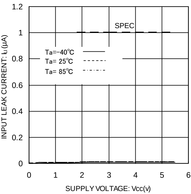
Figure 8. 入力リーク電流 I_L (A0,A1,A2,SCL,WP)
