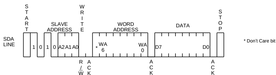
Figure 36. バイトライトサイクル
