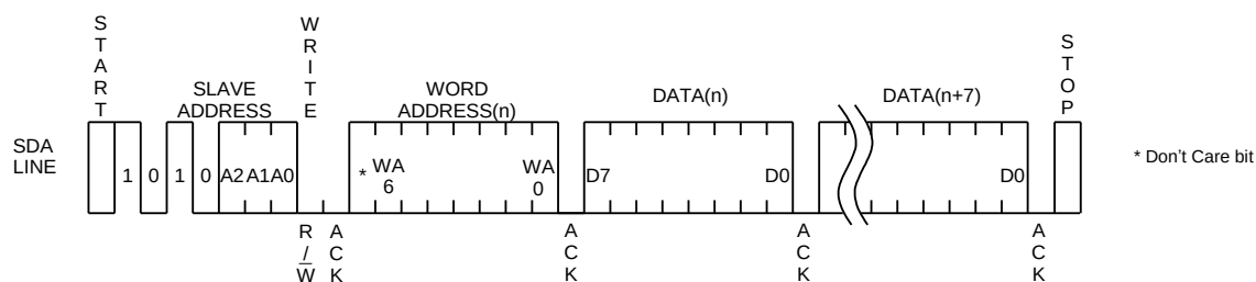
Figure 37. ページライトサイクル
