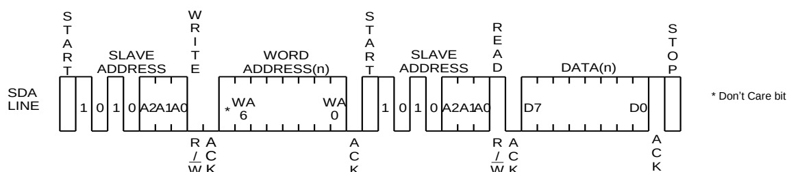
Figure 38. ランダムリードサイクル
