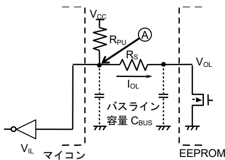
Figure 54. I/O 回路図
