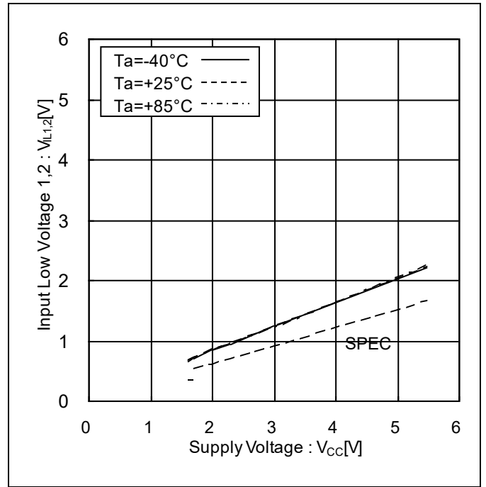
Figure 7. 'LOW'入力電圧 1,2 vs 電源電圧
