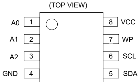
Figure 3-(a). 端子配置図 (SOP8 *1 、SOP-J8、TSSOP-B8、MSOP8) *1 Last Time Buy.
