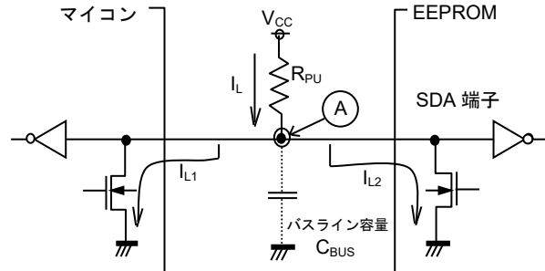
Figure 51. I/O 回路図
