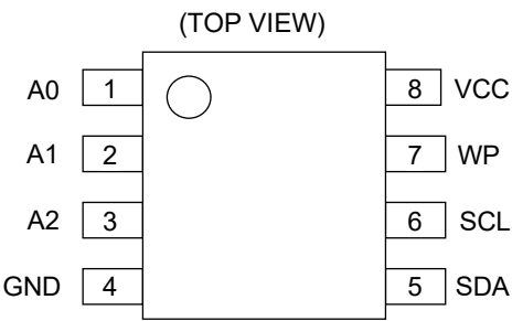
Figure 3. 端子配置図
