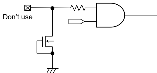
Figure 57. 入力端子回路図 (A0)
