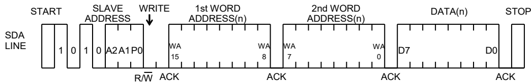
Figure 41. バイトライト
