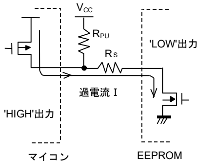
Figure 55. I/O 回路図
