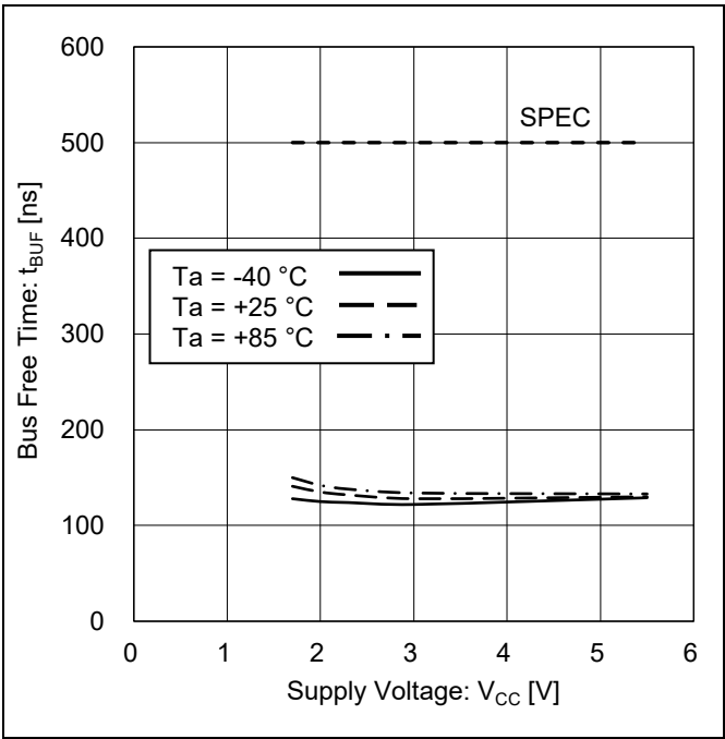
Figure 31. バス開放時間 vs 電源電圧
