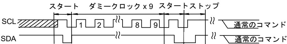
Figure 47. ソフトウェアリセット入力タイミング
