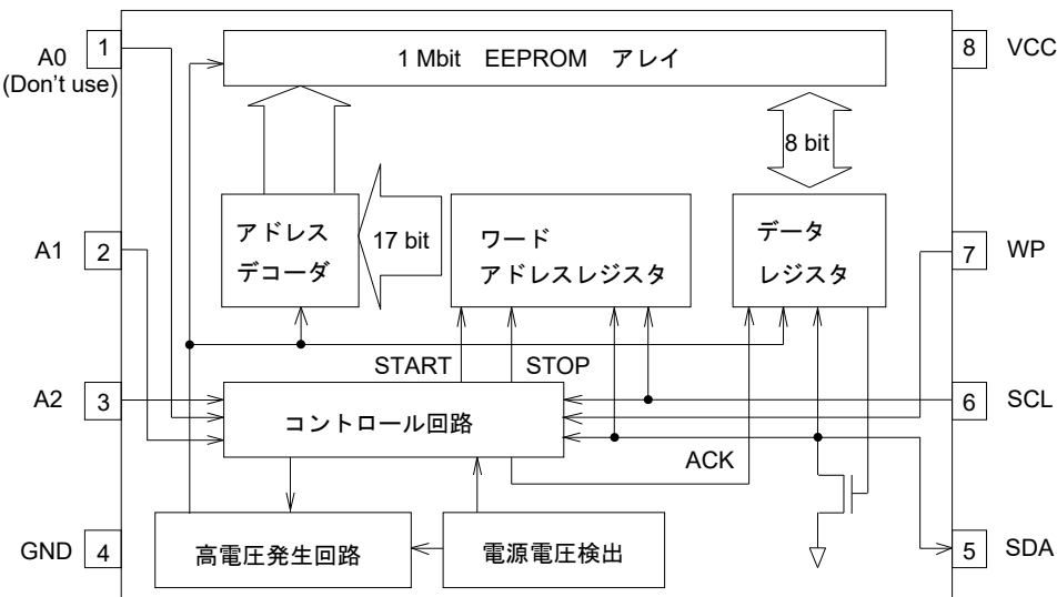
Figure 4. ブロック図
