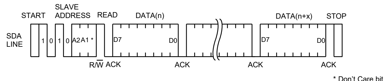
Figure 46. シーケンシャルリード (カレントリードの場合)
