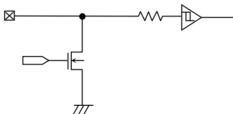
Figure 60. 入出力端子回路図 (SDA)
