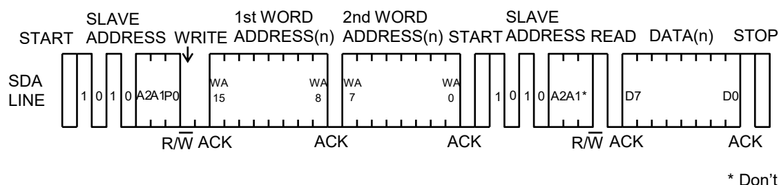
Figure 44. ランダムリード
