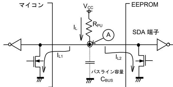
Figure 51. I/O 回路図
