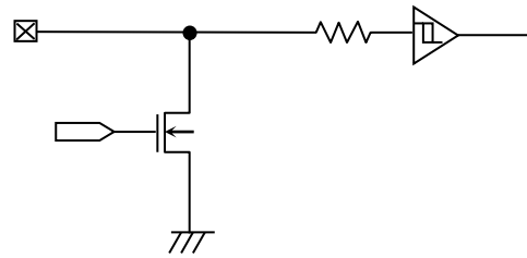
Figure 61. 入出力端子回路図 (SDA)
