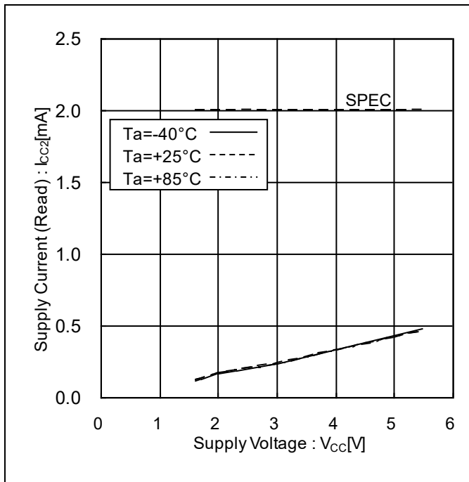
Figure 14. 消費電流(リード) vs 電源電圧 (f CL =1MHz)
