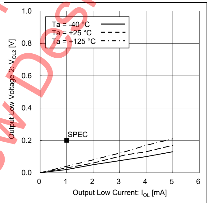
Figure 9. 'LOW'出力電圧 2 vs 'LOW'出力電流 (V CC = 1.7 V)
