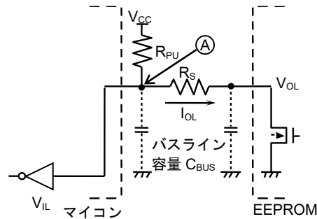
Figure 54. I/O 回路図
