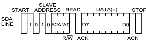
Figure 45. カレントリード
