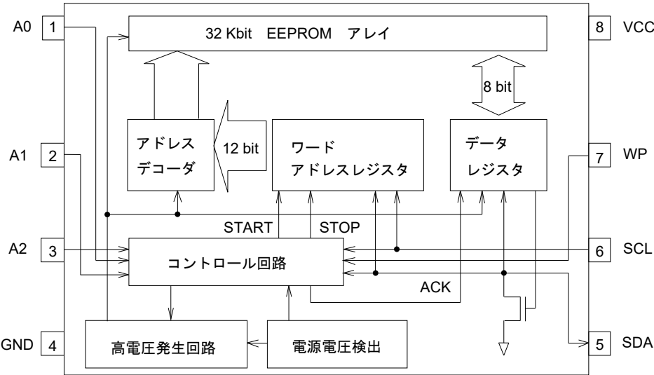
Figure 4. ブロック図
