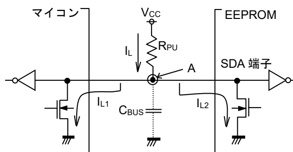
Figure 51. I/O 回路図
