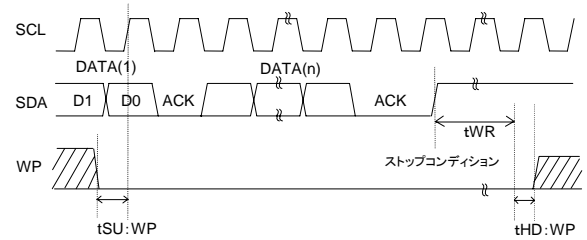
Figure 1-(d) ライト実行時 WP タイミング
