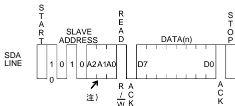
Figure 44. カレントリードサイクル
