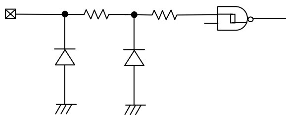
Figure 58. 入力 pin 回路図
