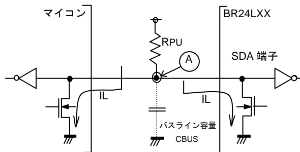
Figure 51. I/O 回路図
