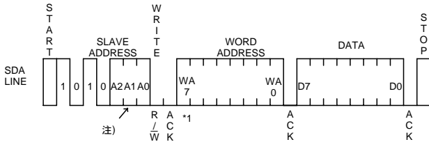
Figure 35. バイトライトサイクル (BR24L01A/02/04/08/16-W)
