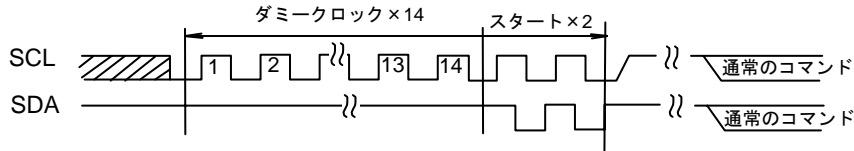
Figure 47-(a) ダミークロック+START+START+コマンド入力の場合
