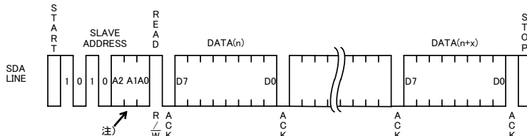
Figure 45. シーケンシャルリードサイクル (カレントリードサイクルの場合)
