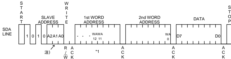
Figure 36. バイトライトサイクル (BR24L32/64-W)
