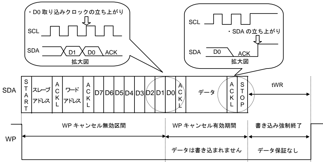
Figure 49. WP 有効タイミング
