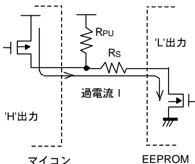
Figure 55. I/O 回路図
