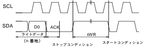
Figure 1-(c) 書き込みサイクルタイミング
