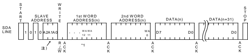
Figure 38. ページライトサイクル (BR24L32/64-W)
