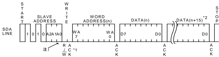
Figure 37. ページライトサイクル (BR24L01A/02/04/08/16-W)
