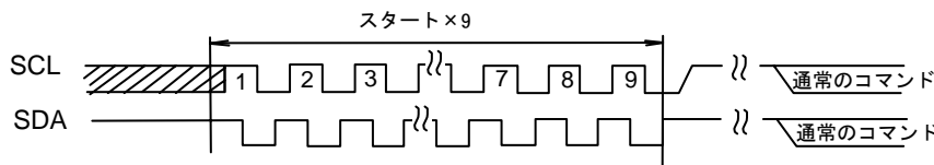
Figure 47-(c) START×9+コマンド入力の場合
