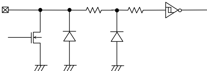
Figure 57. 入出力 pin 回路図
