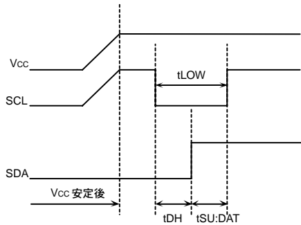
Figure 60. SCL='H' SDA='L'の時
