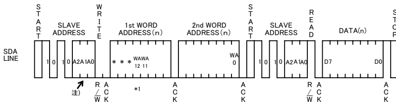
Figure 43. ランダムリードサイクル (BR24L32/64 -W)
