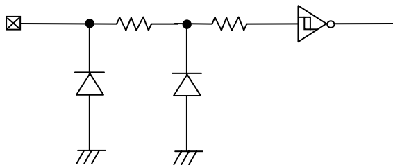
Figure 56. 入力 pin 回路図
