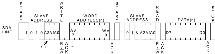
Figure 42. ランダムリードサイクル (BR24L01A/02/04/08/16-W)
