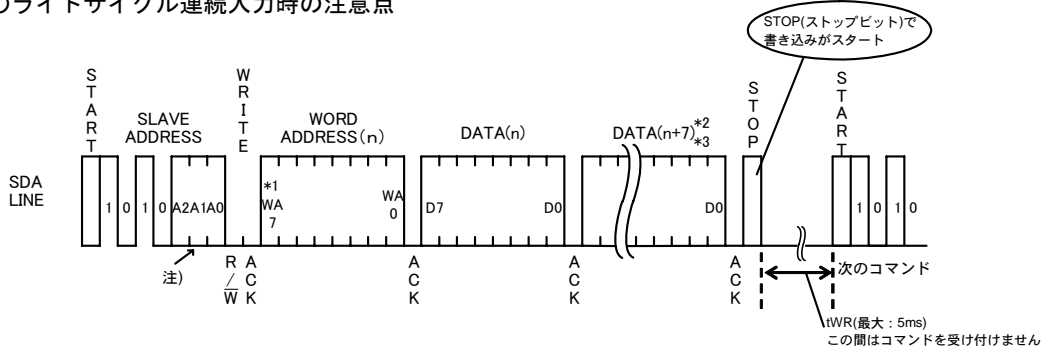
Figure 40. ページライトサイクル
