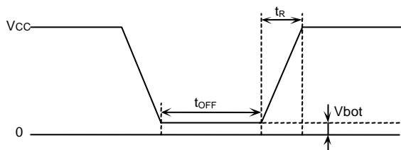
Figure 59. 立ち上がり波形図
