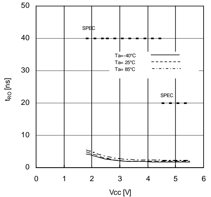
Figure 34. OUTPUT 立ち上がり時間 vs 電源電圧
