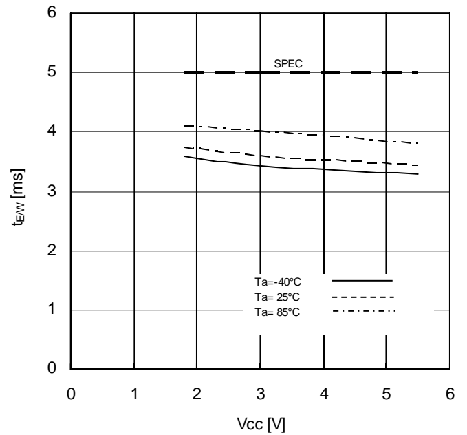
Figure 36. 書き込み時間 vs 電源電圧
