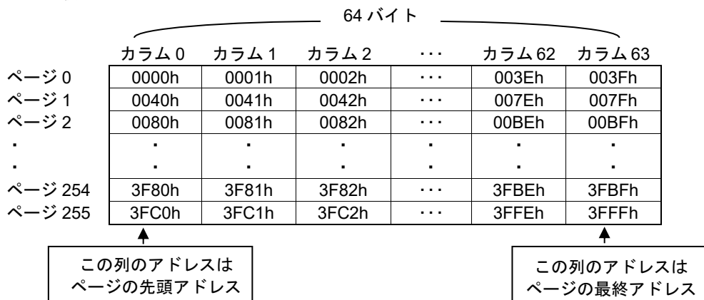
Figure 44. ページライト機能における 64 バイトのページとメモリアレイのアドレスの関係
