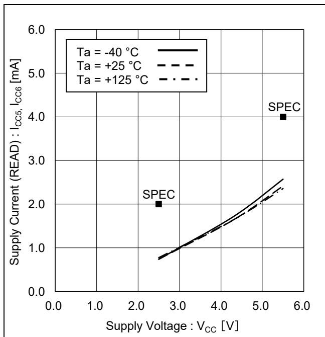
Figure 17. 動作時消費電流 (リード) vs 電源電圧
