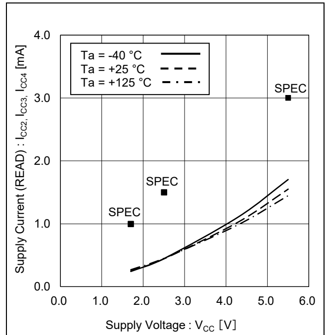
Figure 16. 動作時消費電流 (リード) vs 電源電圧
