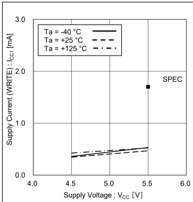
Figure 15. 動作時消費電流 (ライト) vs 電源電圧
