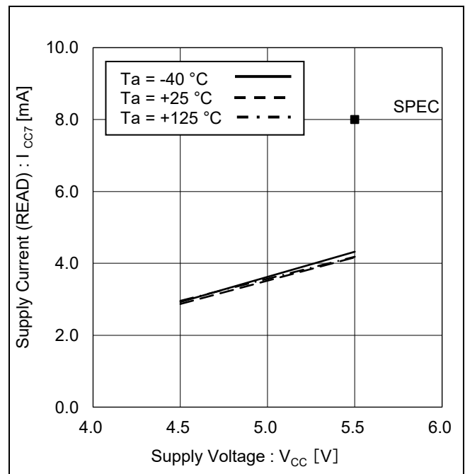
Figure 18. 動作時消費電流 (リード) vs 電源電圧
