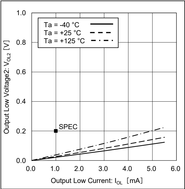
Figure 10. 'LOW'出力電圧 2 vs 'LOW'出力電流 (V<sub>CC</sub> = 1.7 V)
