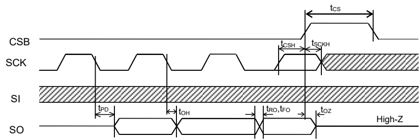
Figure 6-(b). 入出力タイミング
