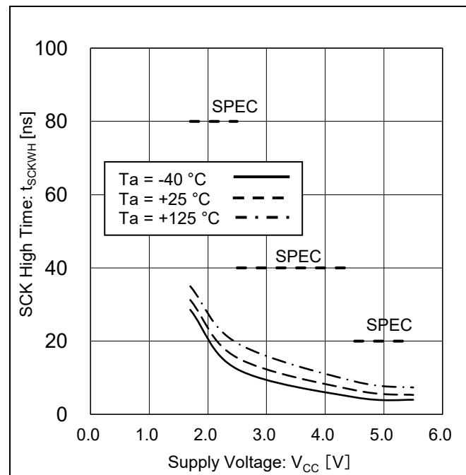
Figure 21. SCK ハイ時間 vs 電源電圧
