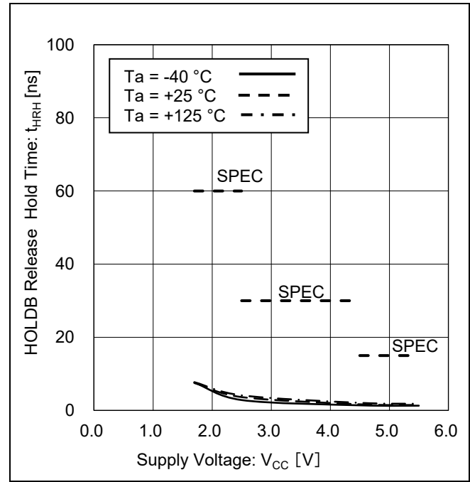
Figure 31. HOLD 解除ホールド時間 vs 電源電圧
