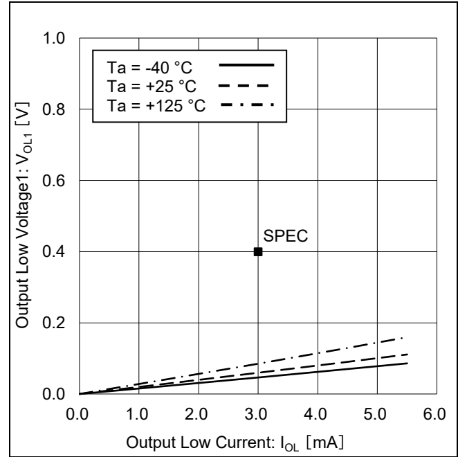
Figure 9. 'LOW'出力電圧 1 vs 'LOW'出力電流 (V<sub>CC</sub> = 2.5 V)
