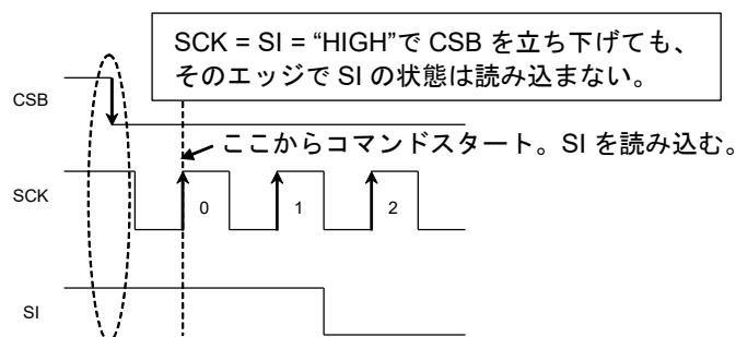
Figure 51. 動作タイミング
