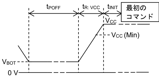
Figure 62. 電源立ち上げ波形図
