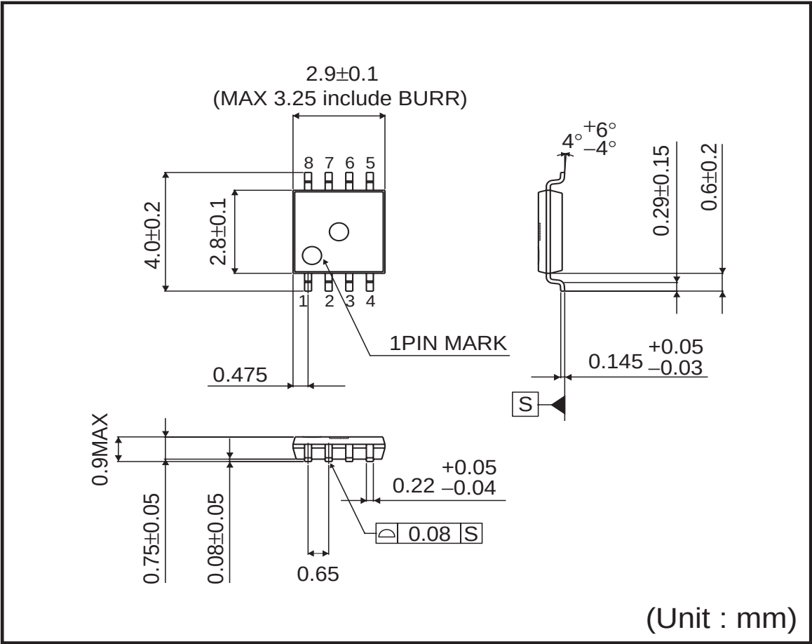
MSOP8
