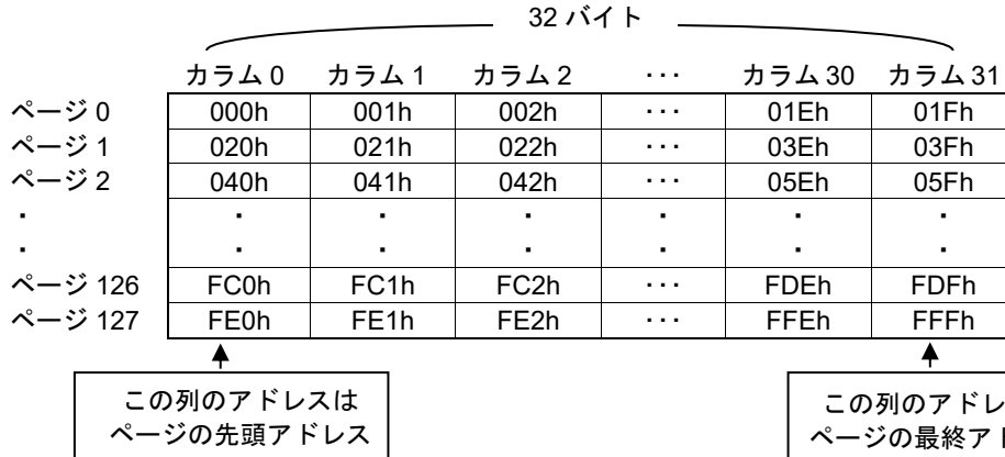
Figure 44. ページライト機能における 32 バイトのページとメモリアレイのアドレスの関係
