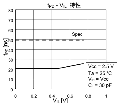
Figure 59. データ出力遅延時間 t_{PD} の V_{IL} 依存性
