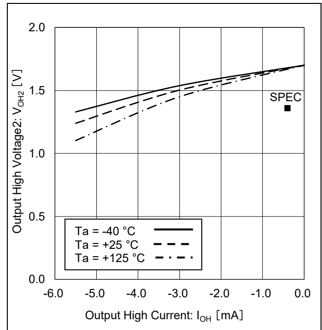
Figure 12. 'HIGH'出力電圧 2 vs 'HIGH'出力電流 ( V_{CC} = 1.7\text{ V} )
