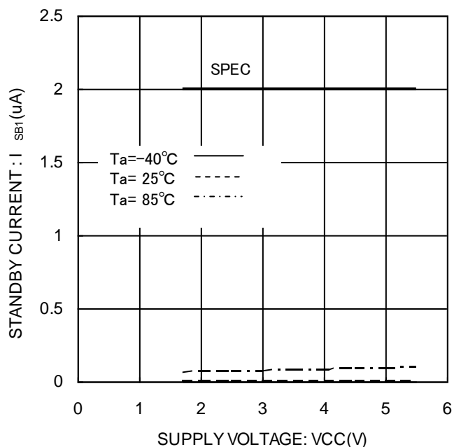
Figure 19. スタンバイ電流 1 I SB1 (CS=0V, ORG=VCC or OPEN)
