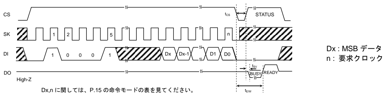
Figure 37. 全アドレス書き込みサイクル
