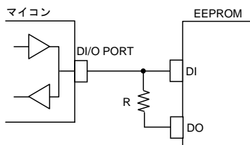
Figure 49. DI, DO 制御ライン共用接続
