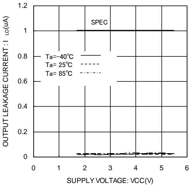
Figure 12. 出力リーク電流 I LO (DO)
