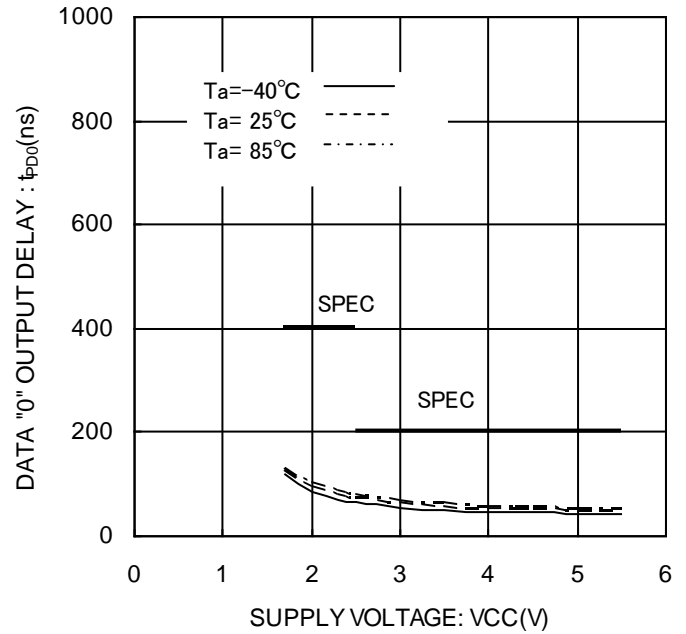
Figure 29. データ"0"出力遅延時間 t_{PD0}
