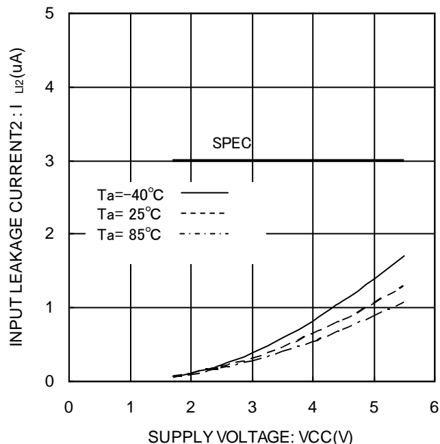
Figure 11. 入力リーク電流 2 I_{L2}(ORG)
