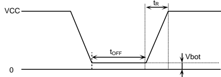
Figure 60. 立ち上がり波形図
