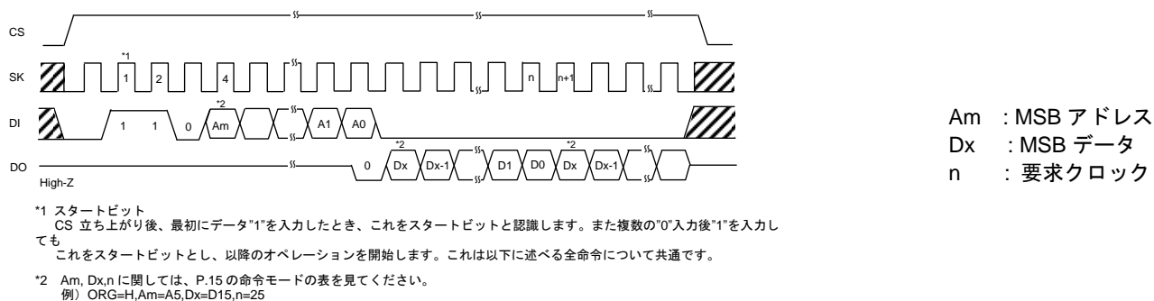
Figure 35. 読み出しサイクル
