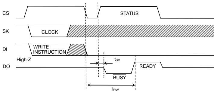
Figure 48. R/B STATUS 出力タイミング図
