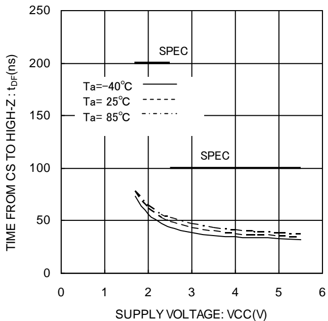
Figure 32. CS より出力 High-Z までの時間 t_{DF}
