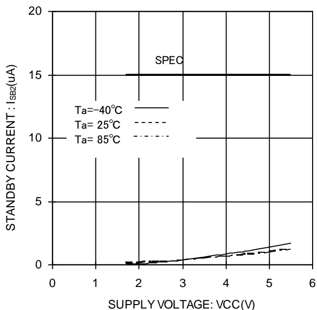
Figure 20. スタンバイ電流 2 I SB2 (CS=0V,DO=OPEN,ORG=0V)
