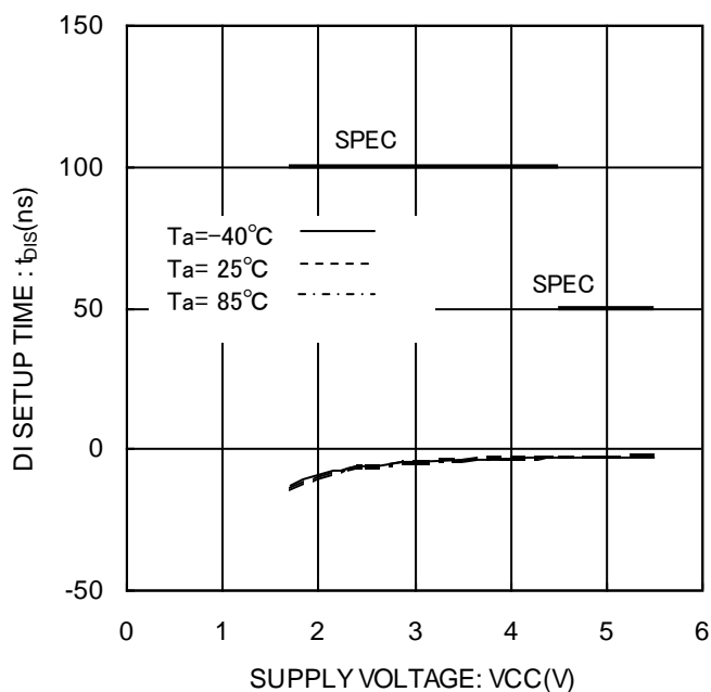
Figure 27. DI セットアップ時間 t_{biS}
