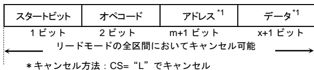
Figure 41. READ キャンセル有効タイミング
