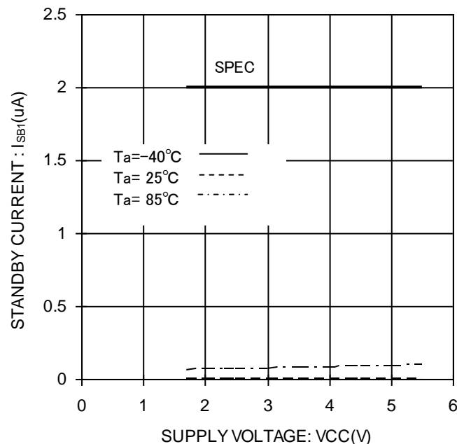
Figure 19. スタンバイ電流 1 I_Sb1(CS=0V, ORG=VCC or OPEN)
