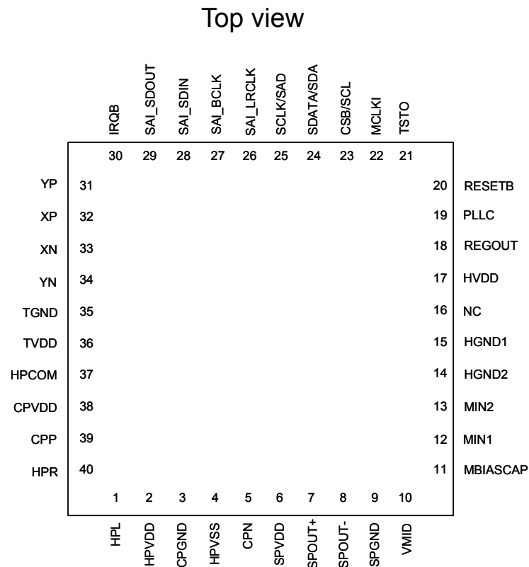
Figure 2. 端子配置図
