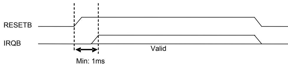
割り込みタイミング Figure 40
