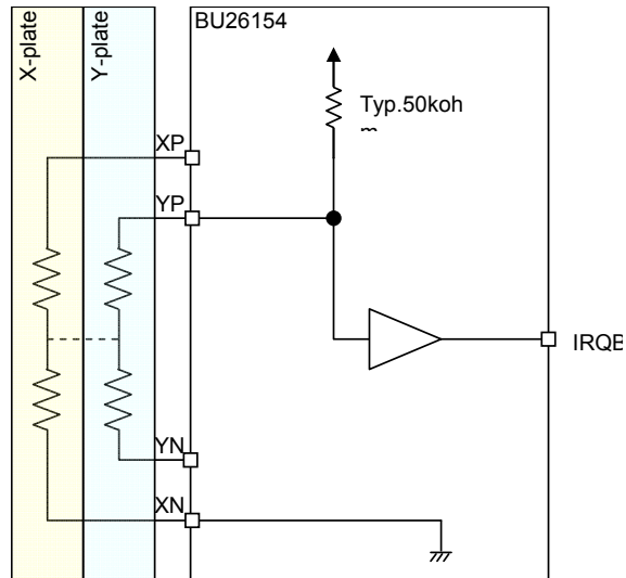
割り込み検出回路 Figure 39
