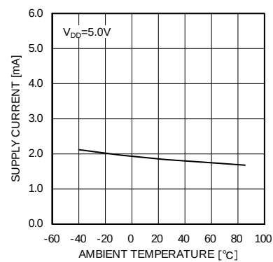
Fig.56 I DD 温度特性
