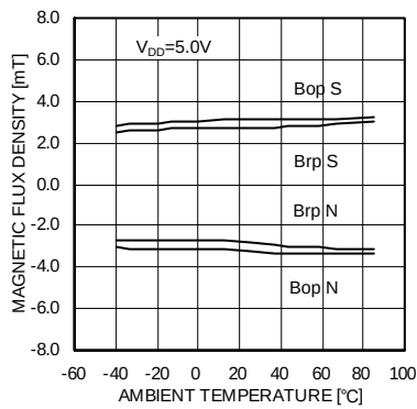
Fig.54 Bop,Brp 温度特性
