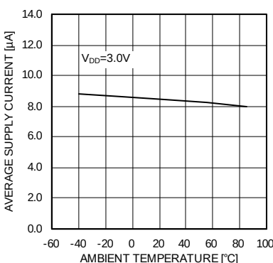
Fig.28 I_{DD} 温度特性
