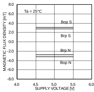
Fig.55 Bop,Brp 電源電圧特性
