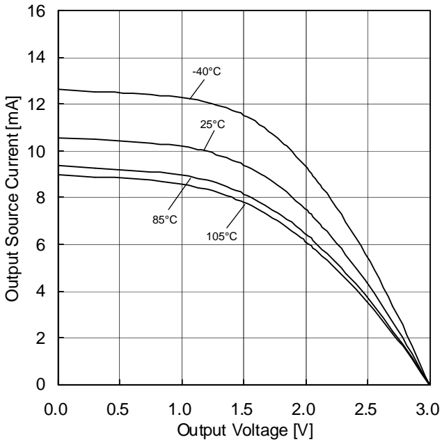
Figure 9. 出カソース電流-出力電圧特性 (VDD=3 V)
