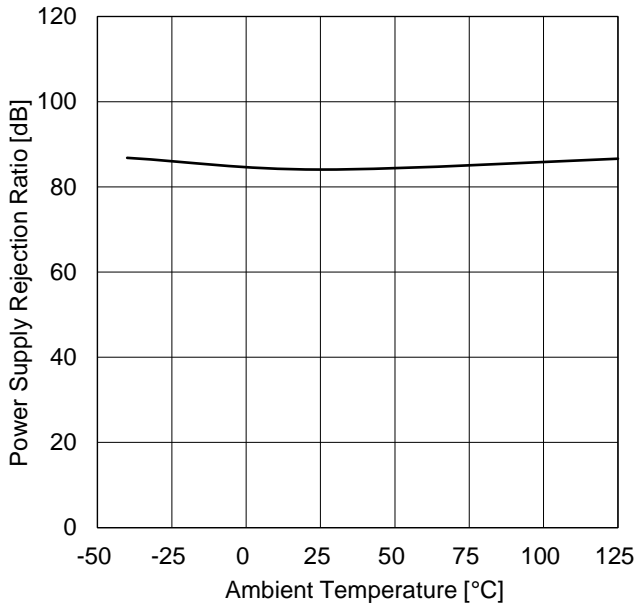
Figure 22. 電源電圧除去比 vs 温度特性
