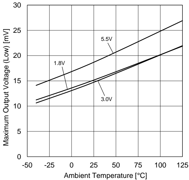
Figure 8. 最大出力電圧(Low) vs 温度特性 ( R_L=10\text{ k}\Omega , V_{RL}=V_{DD} )
