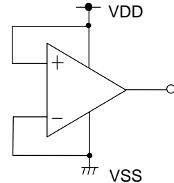
Figure 29. 未使用回路処理例
