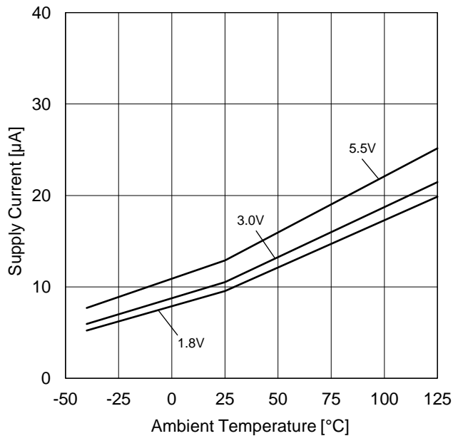
Figure 4. 回路電流 vs 温度特性
