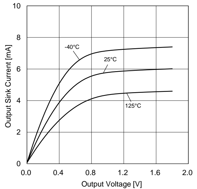
Figure 9. 出力シンク電流 vs 出力電圧特性 ( V_{DD}=1.8\text{ V} )
