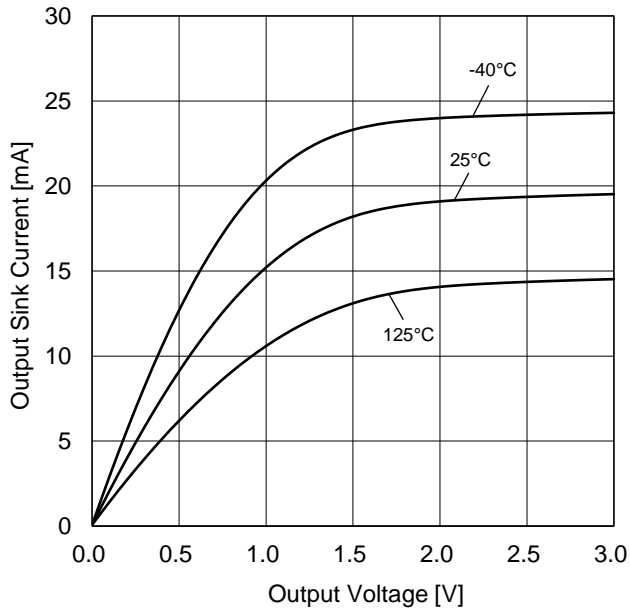
Figure 10. 出力シンク電流 vs 出力電圧特性 (V DD =3 V)
