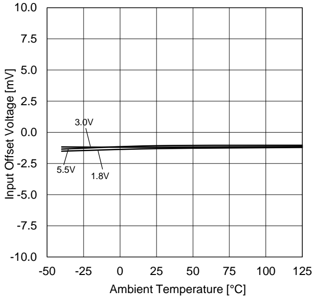
Figure 14. 入力オフセット電圧 vs 温度特性 ( V_{ICM}=V_{DD} , E_K=-V_{DD}/2 )
