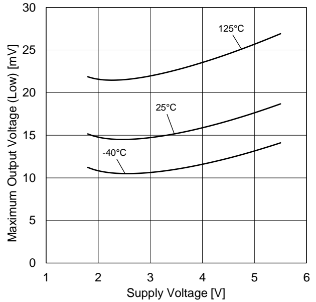
Figure 7. 最大出力電圧(Low) vs 電源電圧特性 ( R_L=10\text{ k}\Omega , V_{RL}=V_{DD} )
