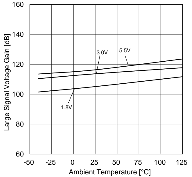
Figure 19. 大振幅電圧利得 vs 温度特性
