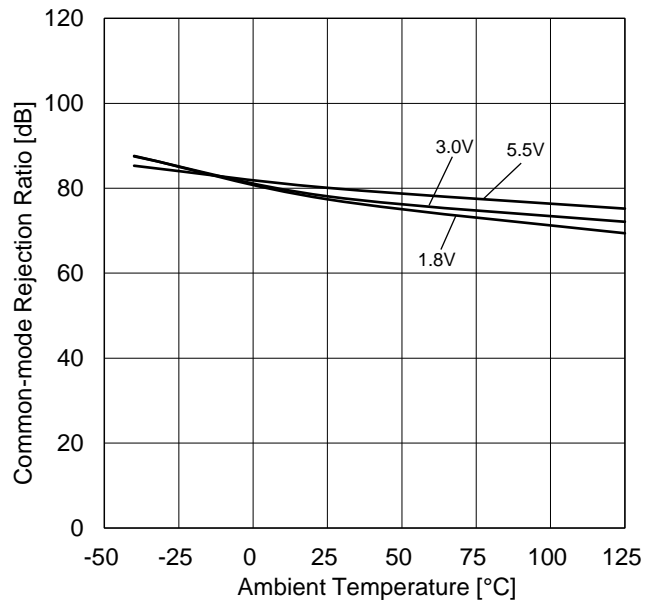
Figure 21. 同相信号除去比 vs 温度特性
