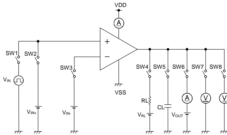
Figure 26. 測定回路2 (1チャンネルのみ)
