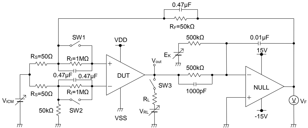
Figure 25. 測定回路 1 (1 チャンネルのみ)
