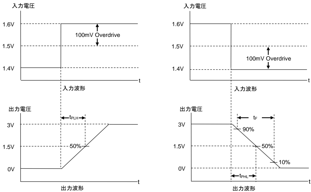
Figure 27. 伝搬遅延時間測定時入出力波形
