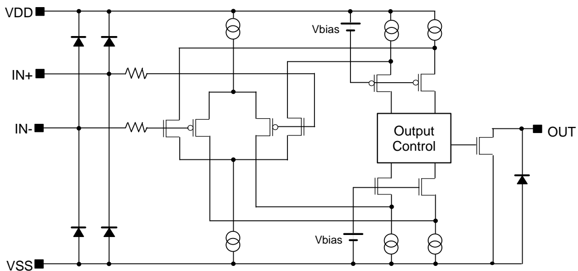
Figure 1. ブロック図 (1チャンネルのみ)
