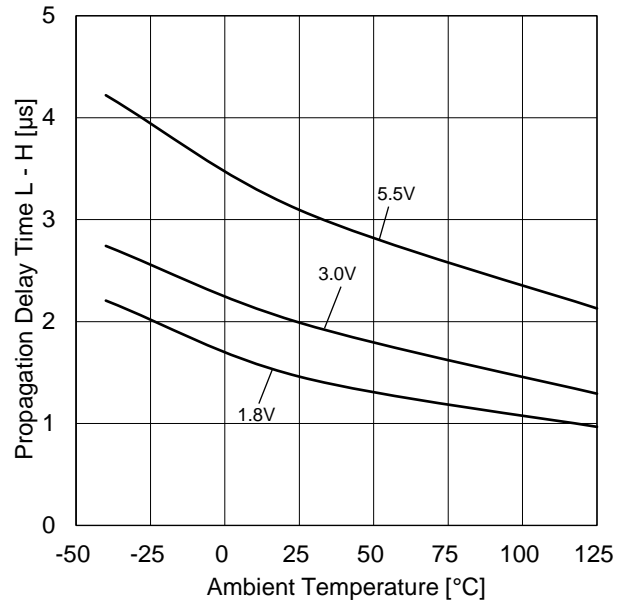
Figure 23. 立ち上がり伝搬遅延時間 vs 温度特性 ( R_L=10\text{ k}\Omega , V_{RL}=3\text{ V} , C_L=15\text{ pF} V_{IN}=1.5\text{ V} , 100 mV Overdrive)
