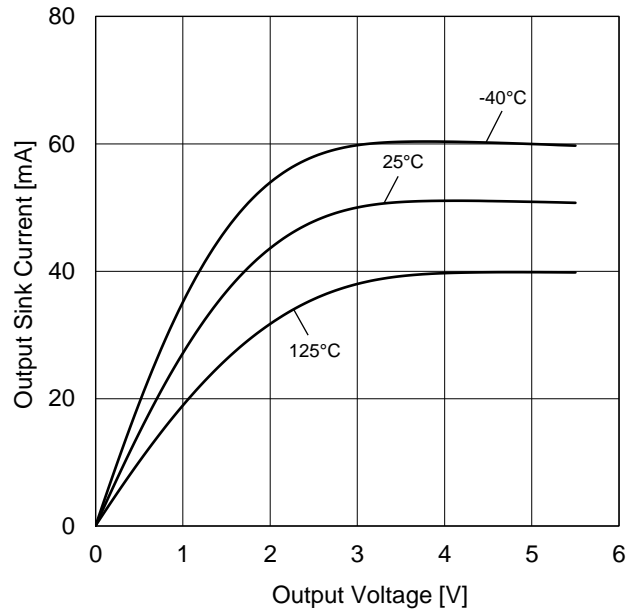
Figure 11. 出力シンク電流 vs 出力電圧特性 (V DD =5.5 V)
