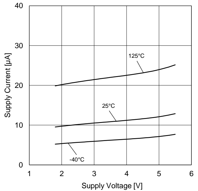
Figure 3. 回路電流 vs 電源電圧特性
