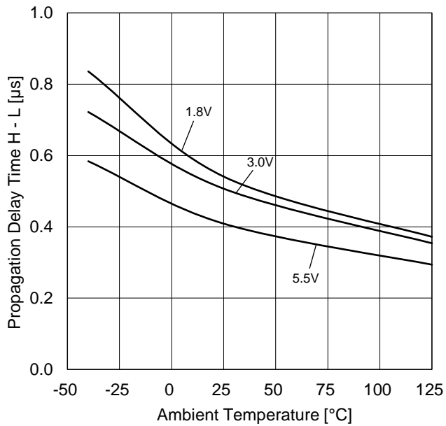
Figure 24. 立ち下がり伝搬遅延時間 vs 温度特性 ( R_L=10\text{ k}\Omega , V_{RL}=3\text{ V} , C_L=15\text{ pF} V_{IN}=1.5\text{ V} , 100 mV Overdrive)
