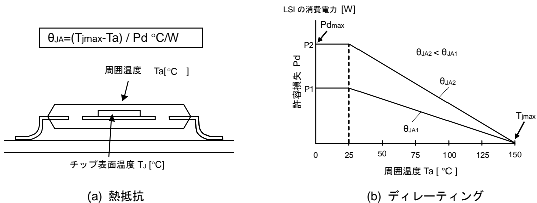
(a) 熱抵抗
