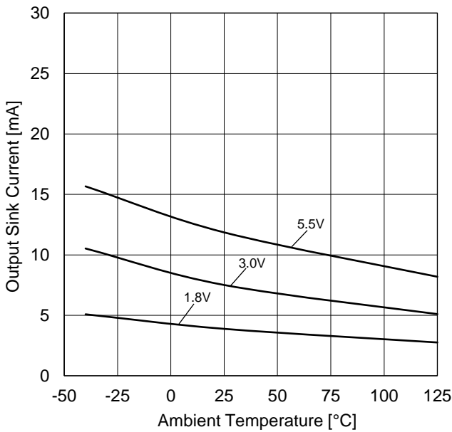
Figure 12. 出力シンク電流 vs 温度特性 (V OUT =V SS +0.4 V)
