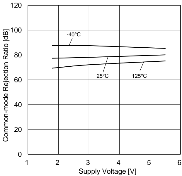
Figure 20. 同相信号除去比 vs 電源電圧特性
