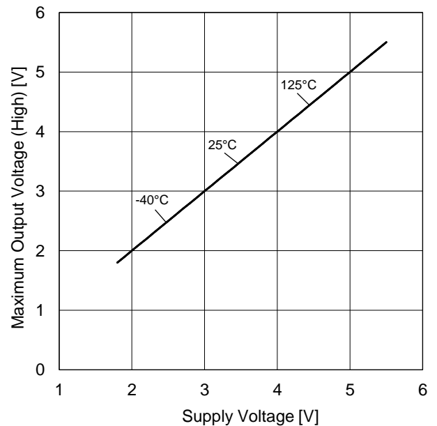
Figure 5. 最大出力電圧(High) vs 電源電圧特性 (RL=10 kΩ, VRL=VDD)
