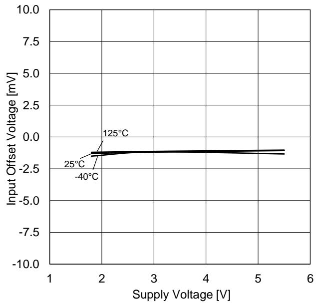
Figure 13. 入力オフセット電圧 vs 電源電圧特性 (V ICM =V DD , E K =-V DD /2)
