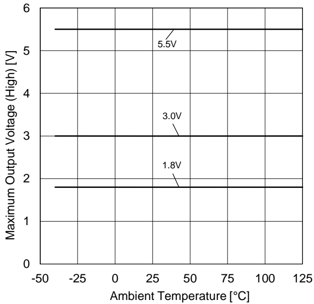
Figure 6. 最大出力電圧(High) vs 温度特性 ( R_L=10\text{ k}\Omega , V_{RL}=V_{DD} )
