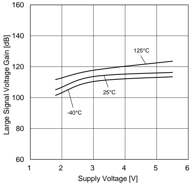
Figure 18. 大振幅電圧利得 vs 電源電圧特性
