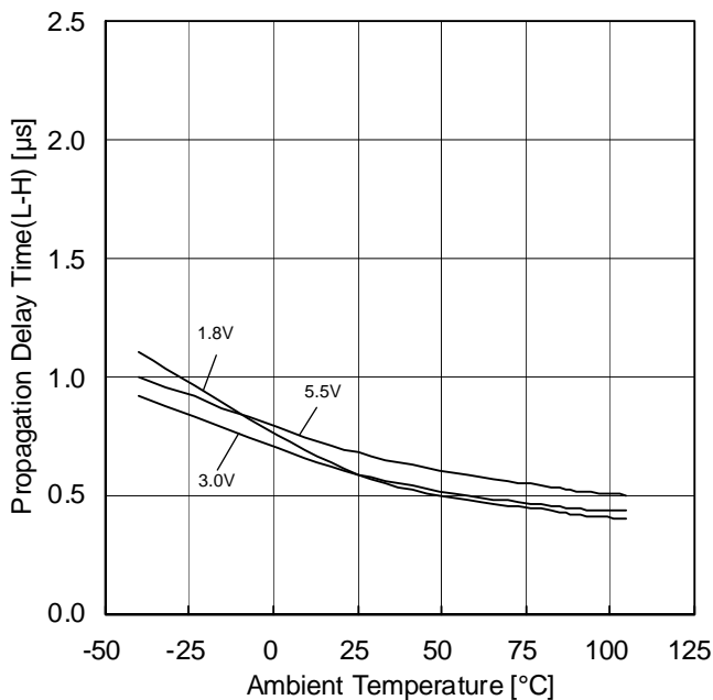
Figure 19. 立ち上がり伝播遅延(L-H)-温度特性 ( R_L=10k\Omega , V_{RL}=3V , C_L=15pF I_N=1.5V , 100mV Overdrive)
