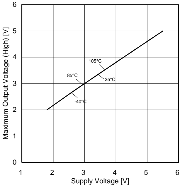
Figure 25. 最大出力電圧(High)－電源電圧特性 ( R_L=10k\Omega )
