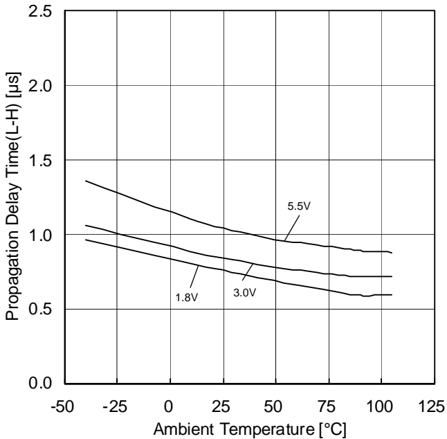
Figure 39. 立ち上がり伝播遅延(L-H)—温度特性 ( R_L=10k\Omega , V_{RL}=3V , C_L=15pF I_N=-1.5V , 100mV Overdrive)
