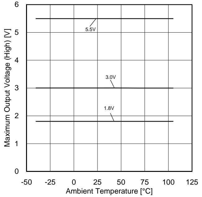
Figure 6. 最大出力電圧(High)－温度特性 ( R_L=10k\Omega , V_{RL}=3V )
