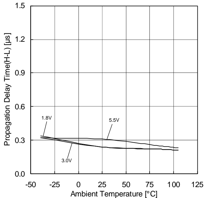
Figure 20. 立ち下がり伝播遅延(H-L)-温度特性 ( R_L=10k\Omega , V_{RL}=3V , C_L=15pF I_N=1.5V , 100mV Overdrive)
