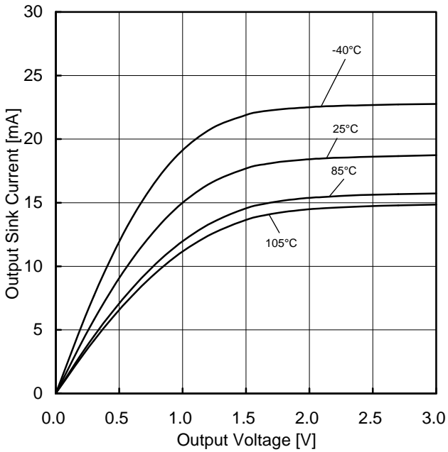
Figure 29. 出力シンク電流－出力電圧特性 (VDD=3 V)
