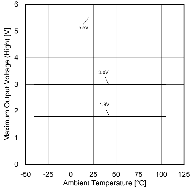
Figure 26. 最大出力電圧(High)－温度特性 ( R_L=10k\Omega )
