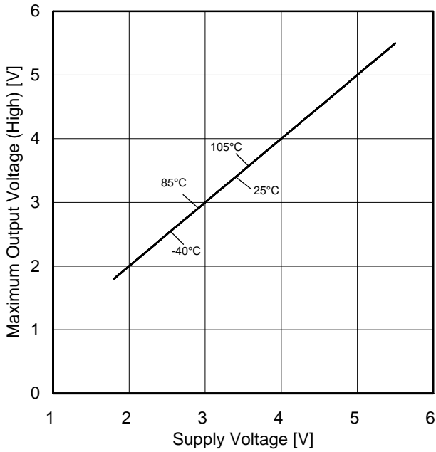
Figure 5. 最大出力電圧(High)－電源電圧特性 ( R_L=10k\Omega , V_{RL}=3V )
