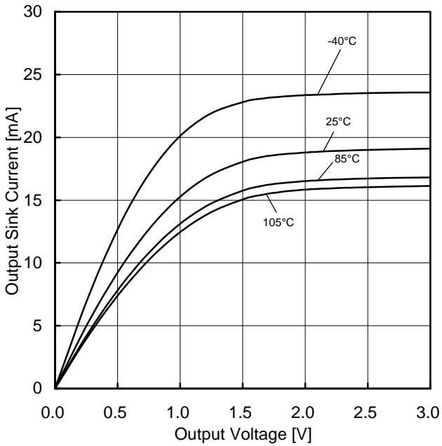
Figure 9. 出力シンク電流—出力電圧特性 (VDD=3 V)
