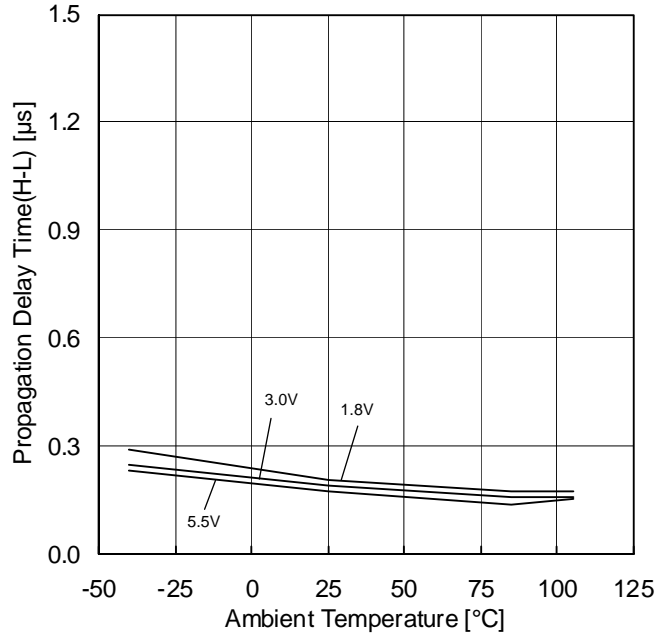
Figure 40. 立ち下がり伝播遅延(H-L)—温度特性 ( R_L=10k\Omega , V_{RL}=3V , C_L=15pF I_N=-1.5V , 100mV Overdrive)
