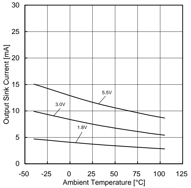
Figure 30. 出力シンク電流－温度特性 (OUT=VSS+0.4V)
