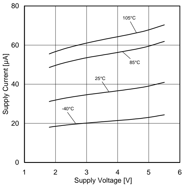
Figure 23. 回路電流 - 電源電圧特性
