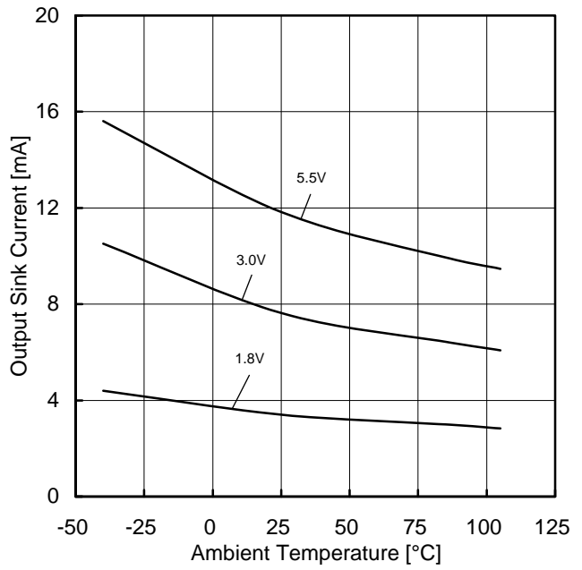
Figure 10. 出力シンク電流—温度特性 (OUT=VSS+0.4V)
