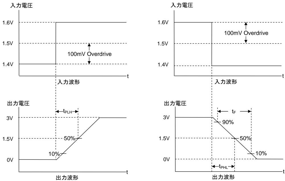
Figure 43. 応答時間測定時 入出力波形
