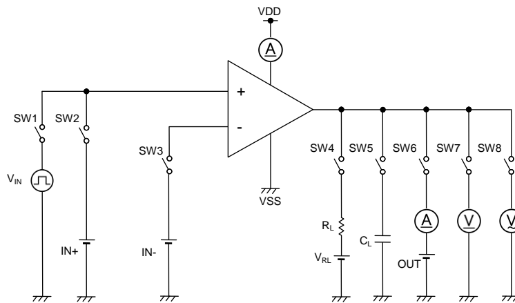
Figure 42. 測定回路 2 (片チャンネルのみ)
