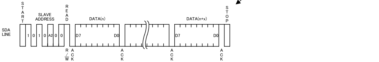
Figure 38. シーケンシャルリードサイクル
