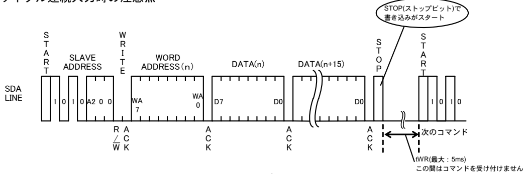
Figure 34. ページライトサイクル
