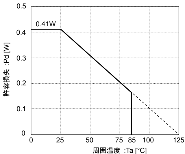
Figure 60. UCSP30L1(BUS1DJC0GWZ / BUS1DJC3GWZ) 許容損失熱軽減特性(参考データ)
