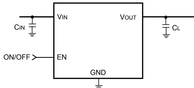
Figure 1. 基本アプリケーション回路
