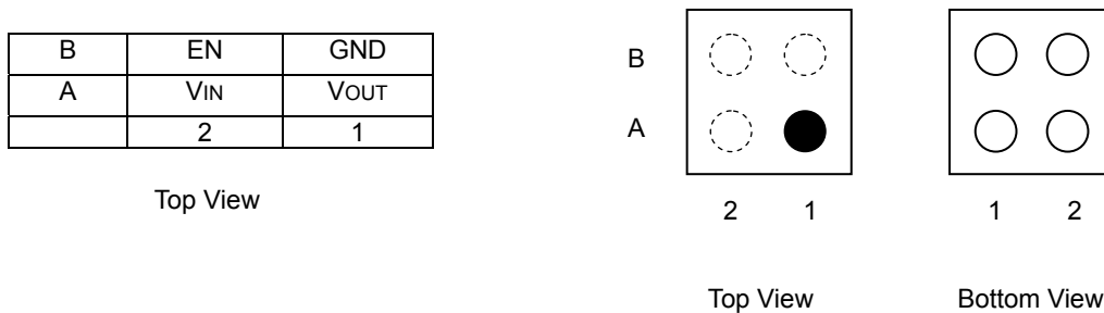
Figure.2 端子配置図
