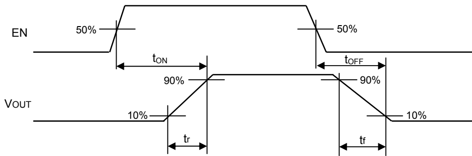
Figure.5 t_{ON}/t_{OFF} 波形
