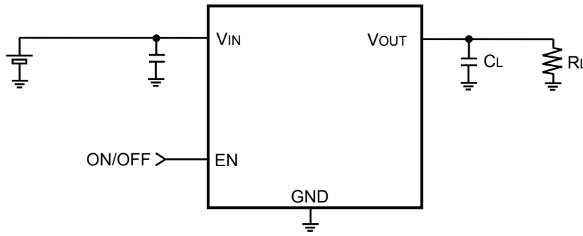
Figure.4 測定回路図
