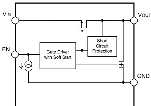
Figure.3 ブロック図
