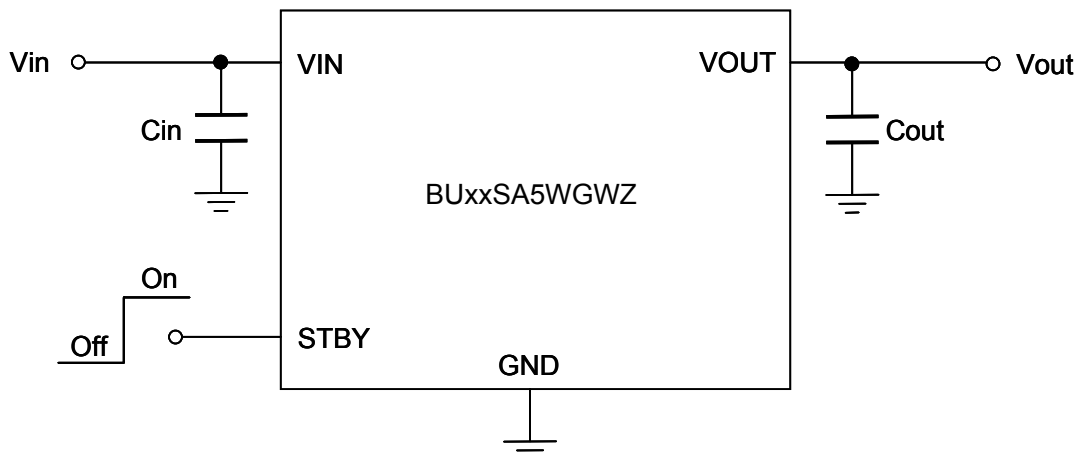
Figure 1. BUxxSA5WGWZ 基本アプリケーション回路図
