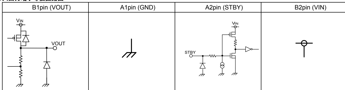
Figure 30. 入出力等価回路
