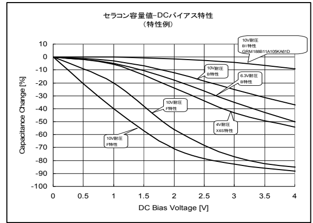
Figure 27. 容量-バイアス特性
