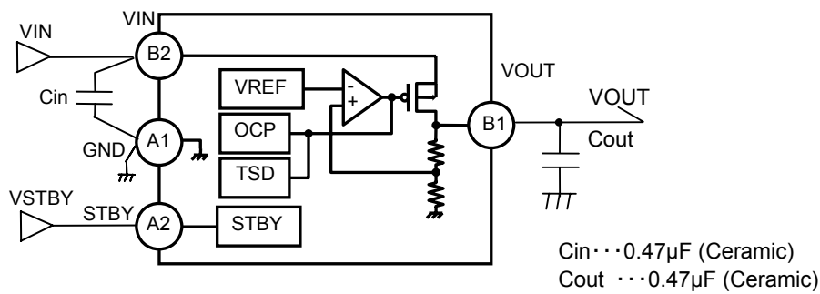
Figure 2. BUxxSA5WGWZ ブロック図
