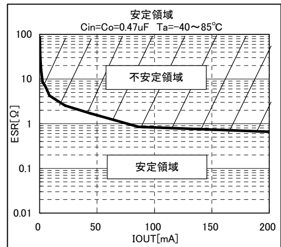
Figure 28. 安定領域特性(特性例)
