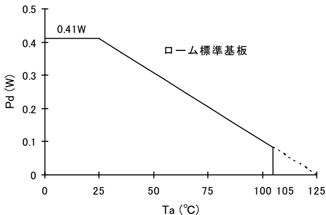
Figure 29. UCSP30L1 (BUXXSA5WGZ) 許容損失熱軽減特性(参考)
