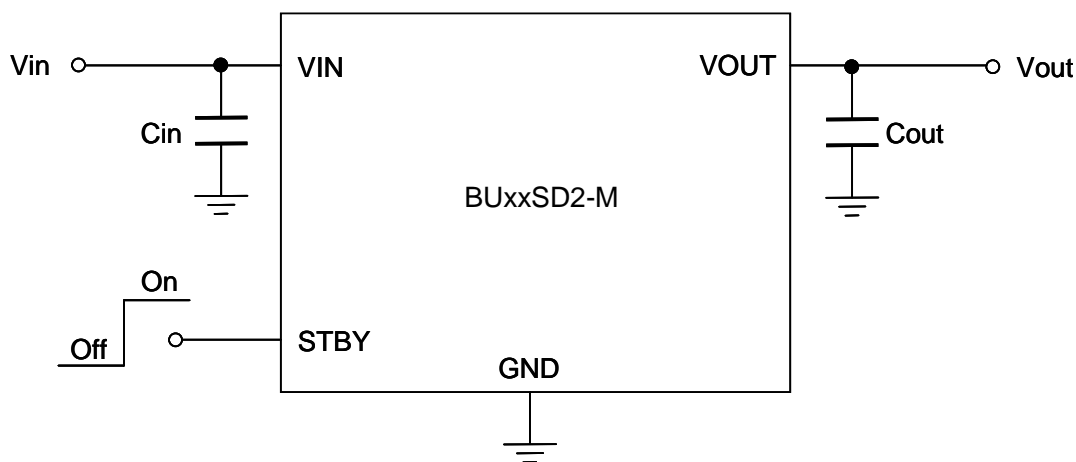
Figure 1. BUxxSD2-M 基本アプリケーション回路図
