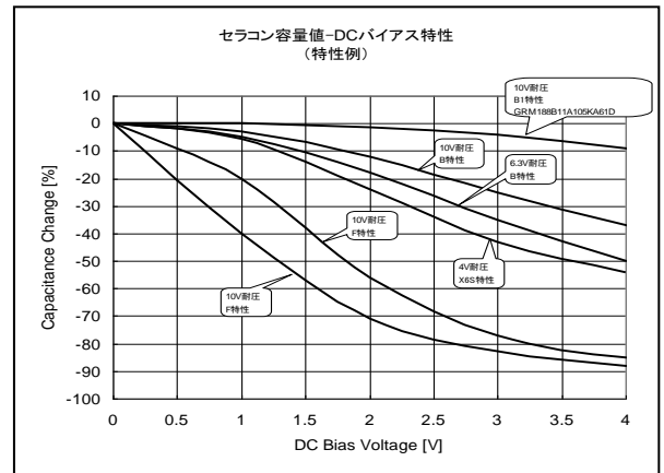
Figure 93. 容量-バイアス特性
