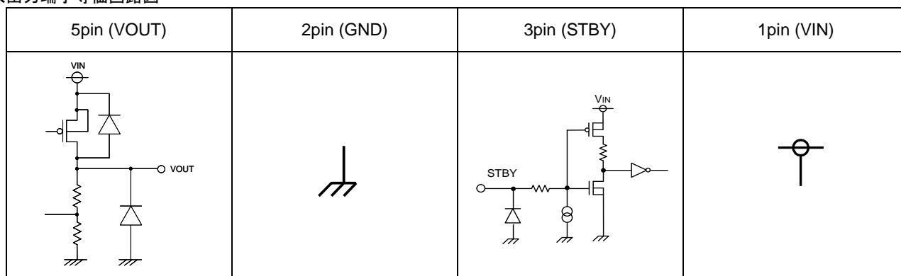
Figure 96. 入出力等価回路
