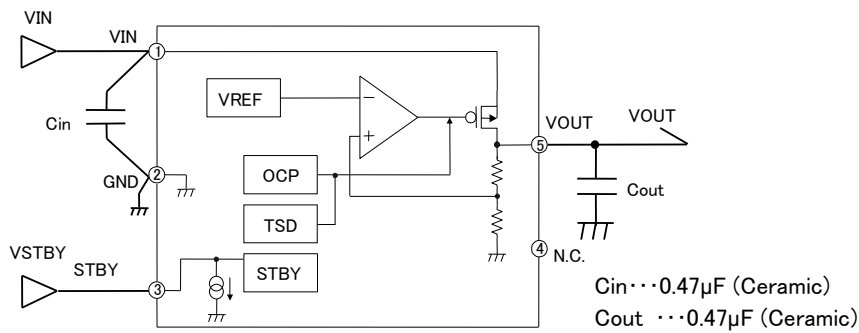
Figure 2. BUxxSD2MG-M ブロック図
