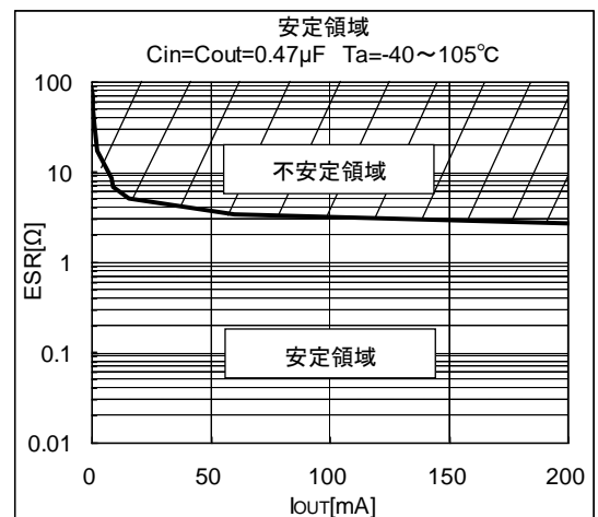
Figure 94. 安定領域特性(特性例)
