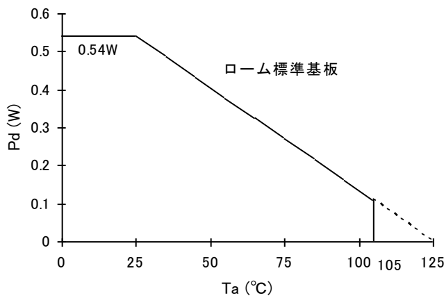
Figure 95. SSOP5 許容損失熱軽減特性(参考)
