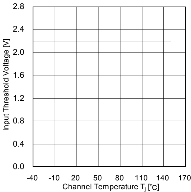
Figure 15. 入力電圧スレッシュヨルド特性[温度特性]
