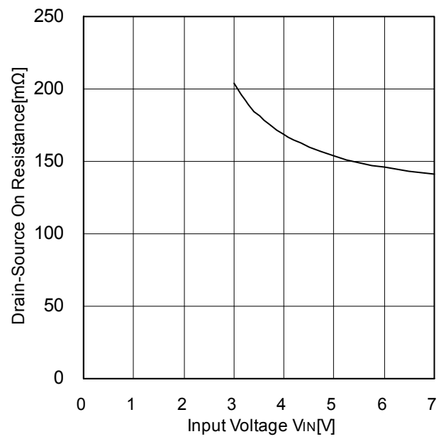
Figure 10. 出力オン抵抗特性[入力電圧特性]
