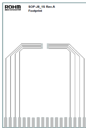
Figure 2. PCB レイアウト 1s (1層)
