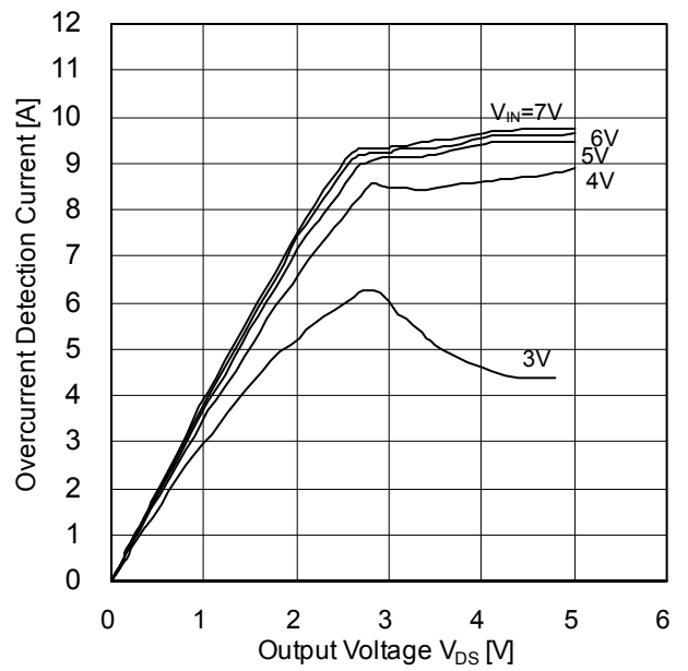
Figure 18. 過電流検出電流特性[入力電圧特性]
