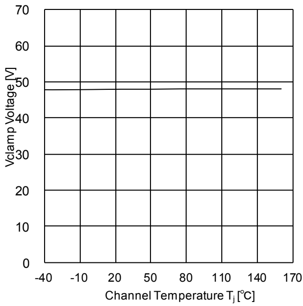
Figure 9. 出力クランプ電圧 vs. ジャンクション温度
