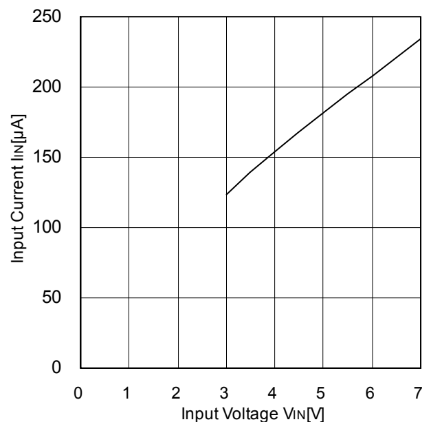
Figure 16. 入力電流特性[入力電圧特性]
