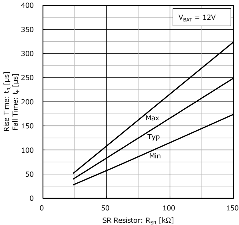
Figure 31. 立ち上がり (立下り) 時間 vs SR 端子抵抗値
