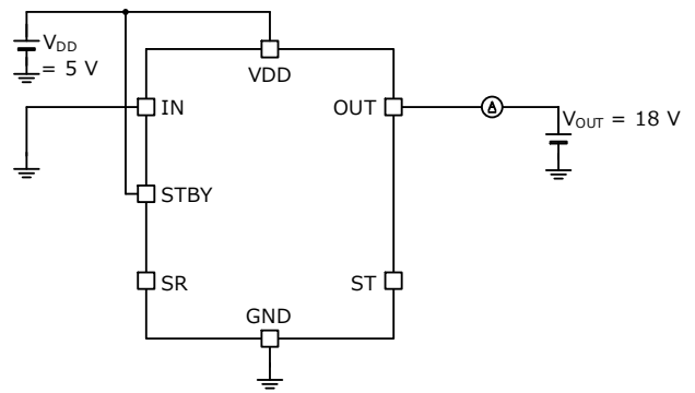
Figure 10、Figure 11 の測定回路図
