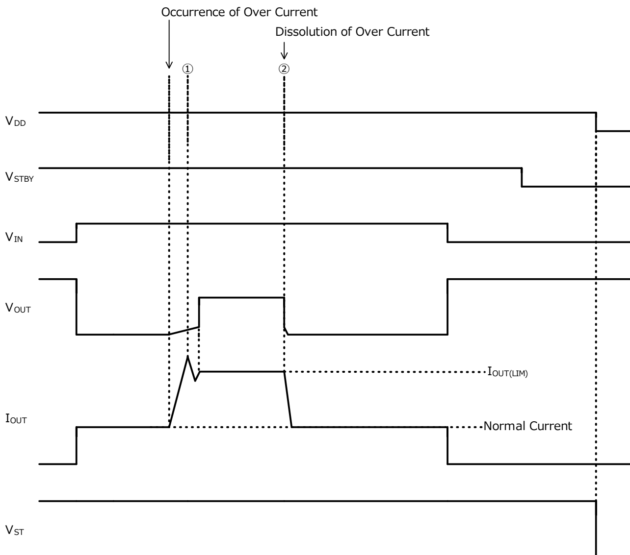
Figure 29. 過電流保護機能のタイミングチャート
