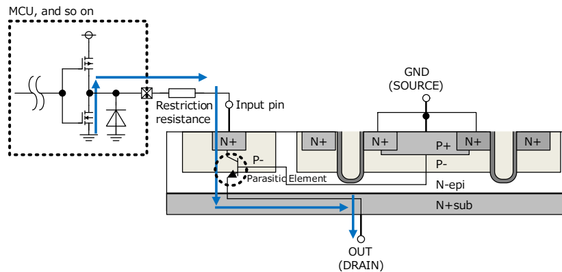
Figure 35. 出力負電流経路(入力端子が Low の場合)
