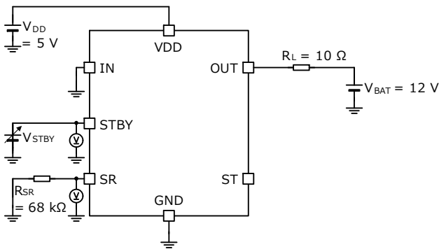
Figure 4 の測定回路図
