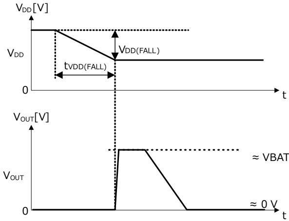
Figure 36. 電源急峻変動時の出力 OFF 動作
