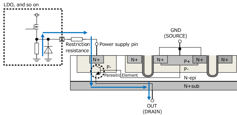
Figure 34. 出力負電流経路(電源端子が Low の場合)
