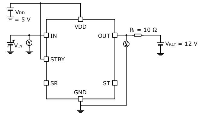
Figure 5 の測定回路図
