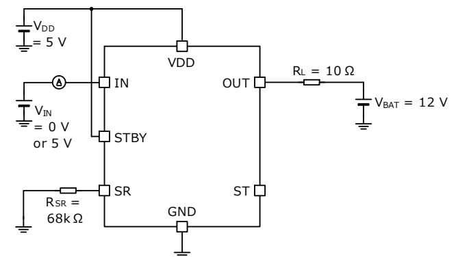
Figure 7 の測定回路図
