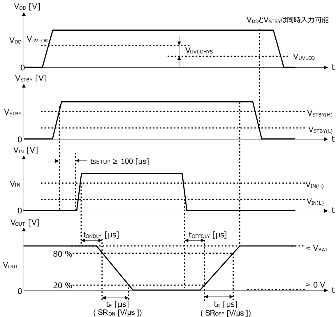
Figure 27. ターンオン時間、ターンオフ時間、立ち下がり時間(スルーレートオン),立ち上がり時間(スルーレートオフ)の定義
