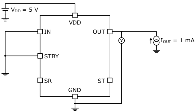
Figure 12 の測定回路図
