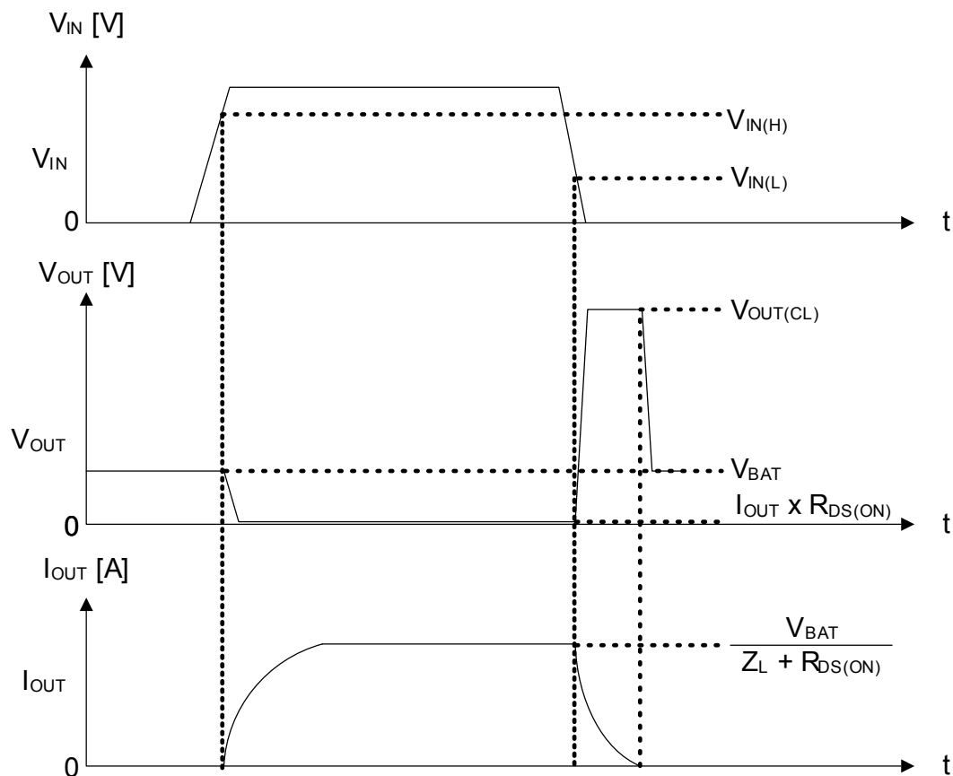
Figure 28. 誘導性負荷時動作
