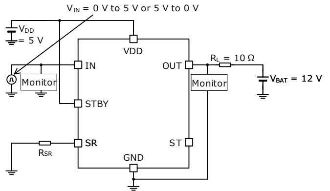
Figure 13、Figure 14、Figure 15、Figure 16、Figure 17、 Figure 18、Figure 19、Figure 20、Figure 21、Figure 22、 Figure 23、Figure 24 の測定回路図
