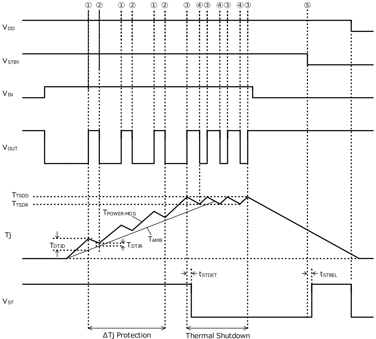
Figure 30. Dual TSD 機能のタイミングチャート
