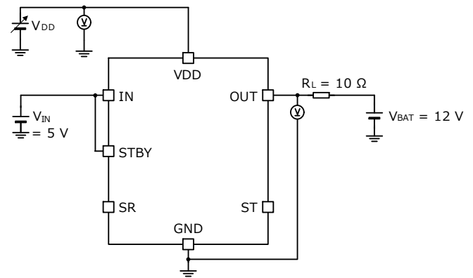
Figure 3 の測定回路図
