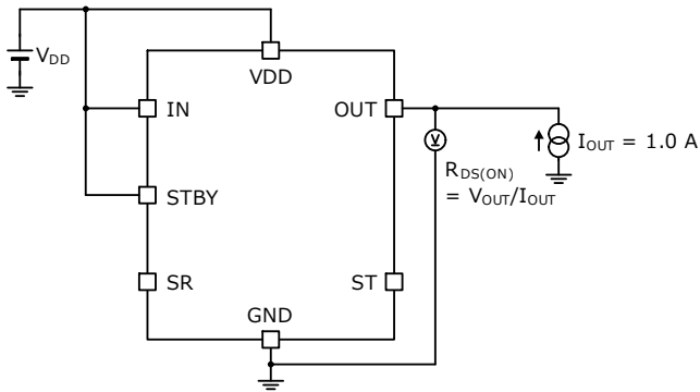
Figure 8、Figure 9 の測定回路図
