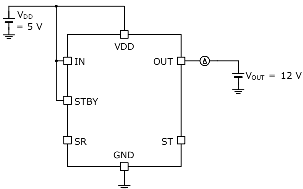
Figure 25 の測定回路図
