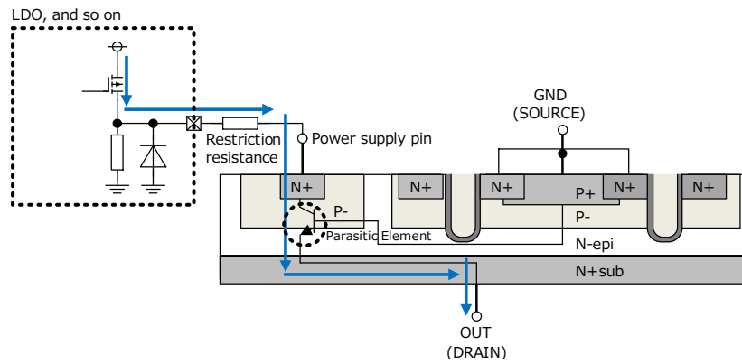
Figure 32. 出力負電流経路(電源端子が High の場合)
