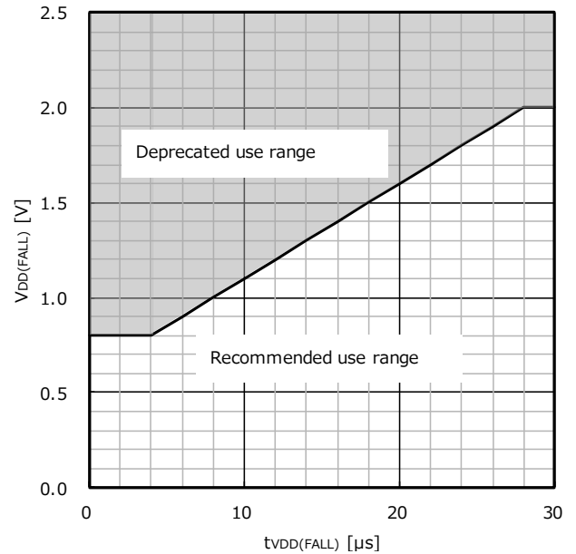
Figure 37. 推奨使用範囲
