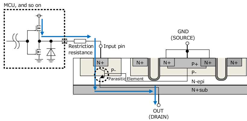
Figure 33. 出力負電流経路(入力端子が High の場合)
