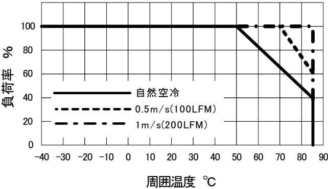
図1 出力デレーティングカーブ
