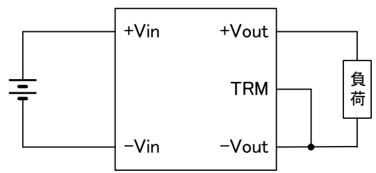
図9 非絶縁で使用する場合の接続
