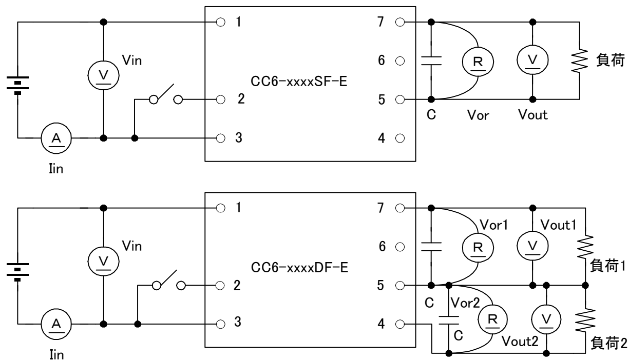
図3 測定回路図
