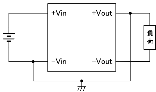
図10 極性反転出力で使用する場合の接続
