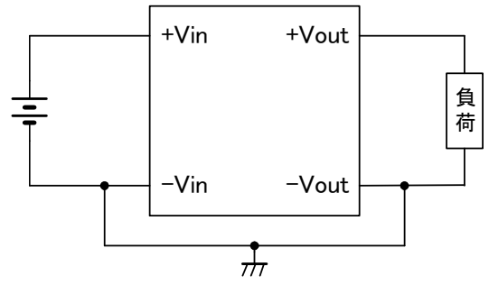
図9 非絶縁で使用する場合の接続
