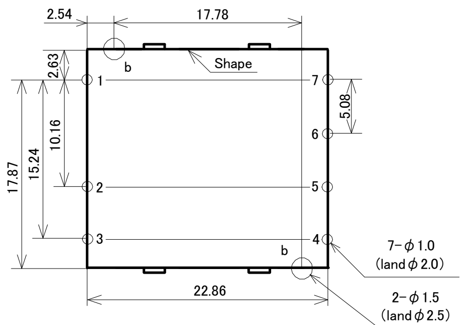
図 12 推奨基板取り付け寸法 (TOP View)
