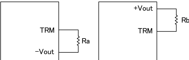
図6 TRM端子抵抗接続方法
