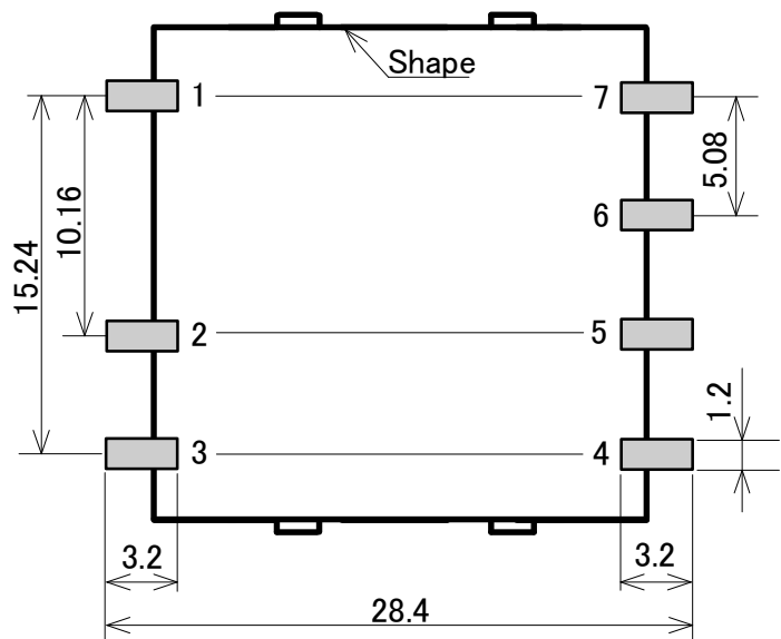
図 13 推奨基板取り付け寸法 (TOP View)
