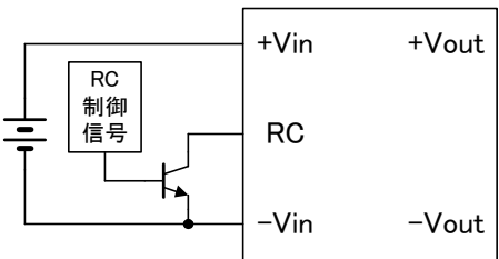
図5 RC端子接続方法
