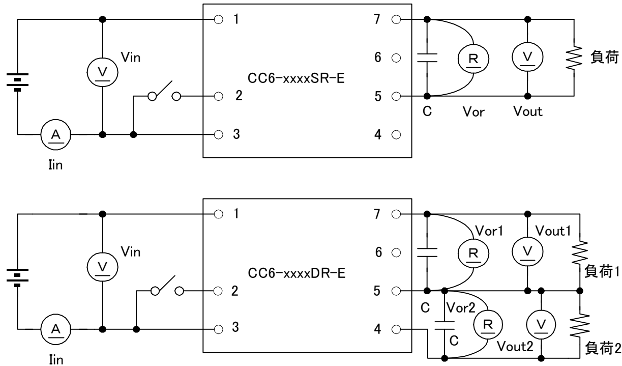
図 3 測定回路図
