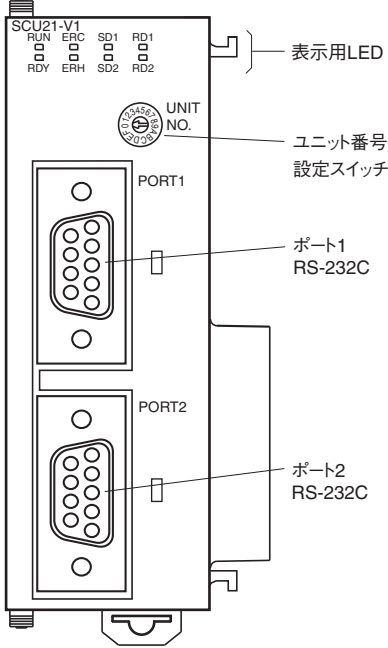
形CJ1W-SCU21-V1/SCU22
