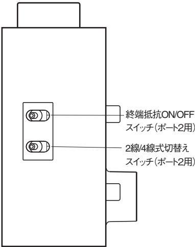
底面図(形CJ1W-SCU3□(-V1)のみ)
