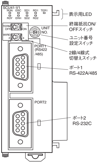
形CJ1W-SCU41-V1
