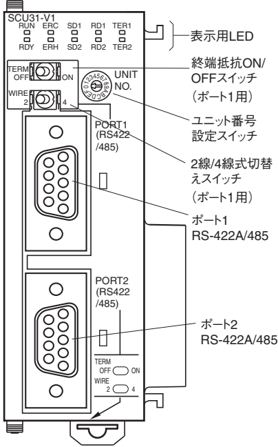
形CJ1W-SCU31-V1
