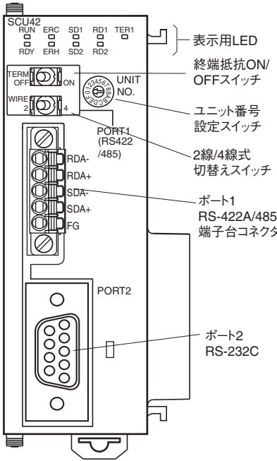
形CJ1W-SCU42
