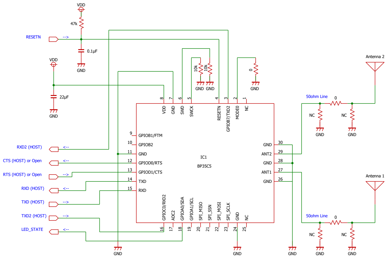
図 2.2. 参考回路図
