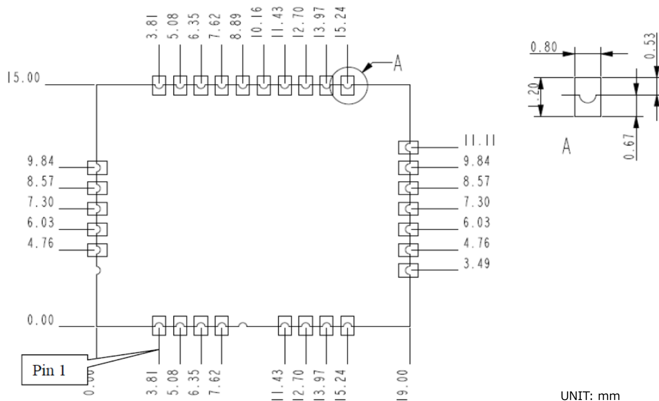
図 5. 推奨ランドパターン図
