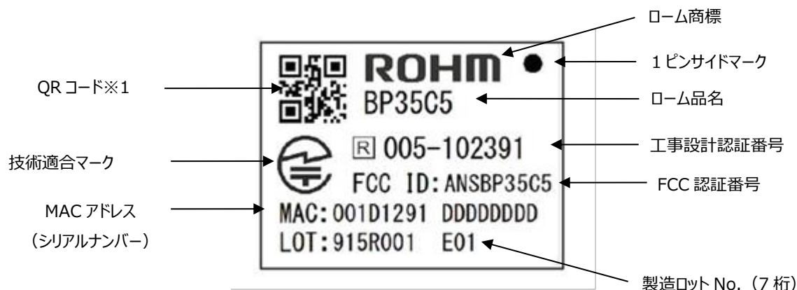
図 4. 標印仕様
