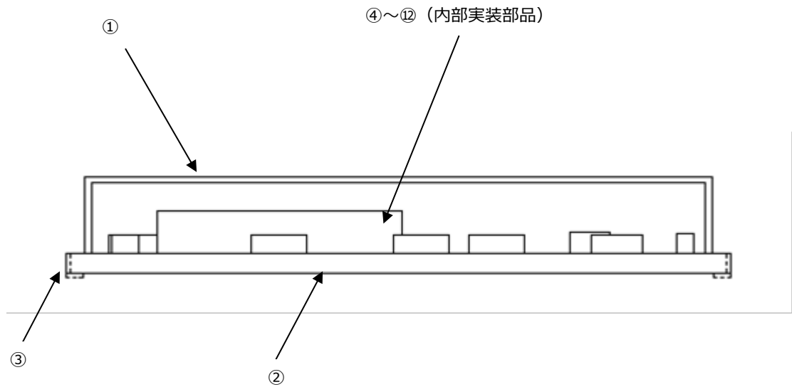
図 6. 内部構造図
