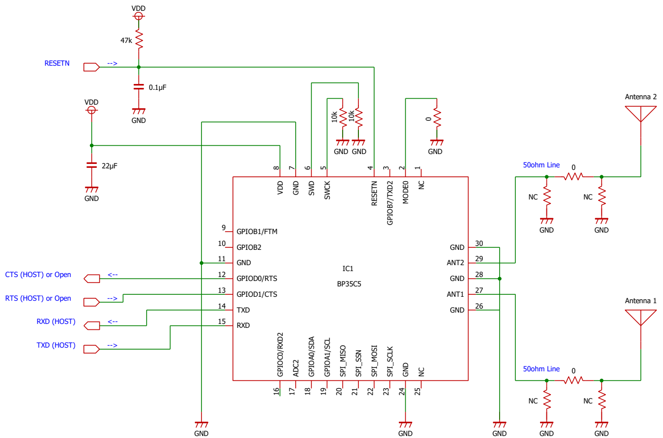
図 2.1. 参考回路図
