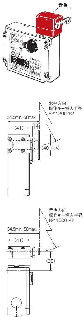
形D4BL+形D4BL-K2の場合
