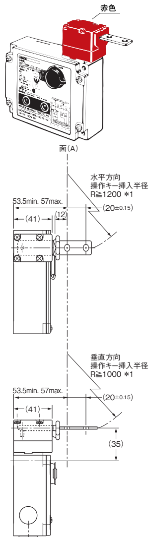
形D4BL+形D4BL-K1の場合
