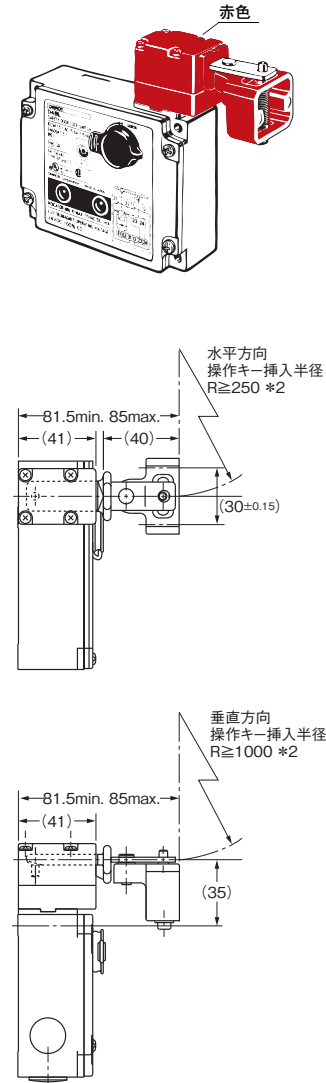
形D4BL+形D4BL-K3の場合
