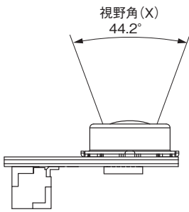
形D6T-44L-06 視野角 (X方向)
