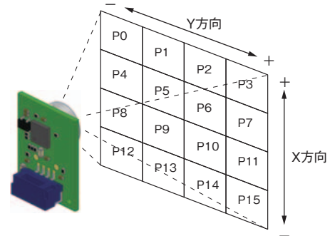
各ピクセルの検出エリア
