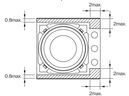
保持・固定可能エリア(斜線部) Top View
