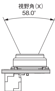
形D6T-1A-02 視野角 (X方向)
