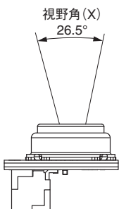
形D6T-1A-02 視野角 (X方向)
