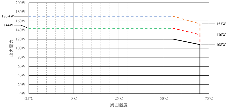
図.13: 標準取付
