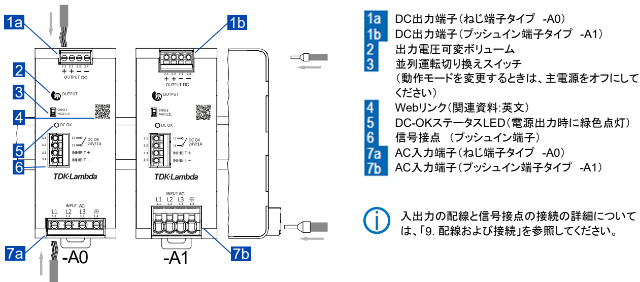
図.1: 端子説明
