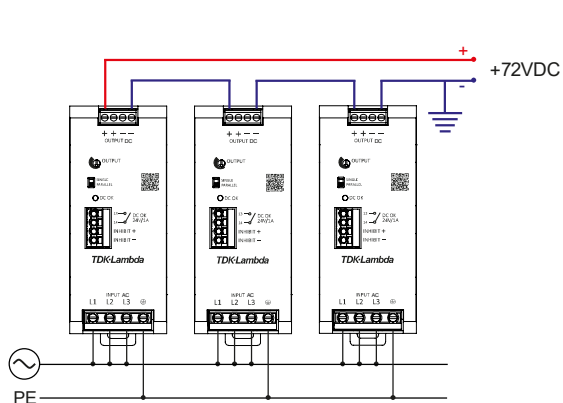
図.34: 正電圧レベルでの直列動作の接続方式
