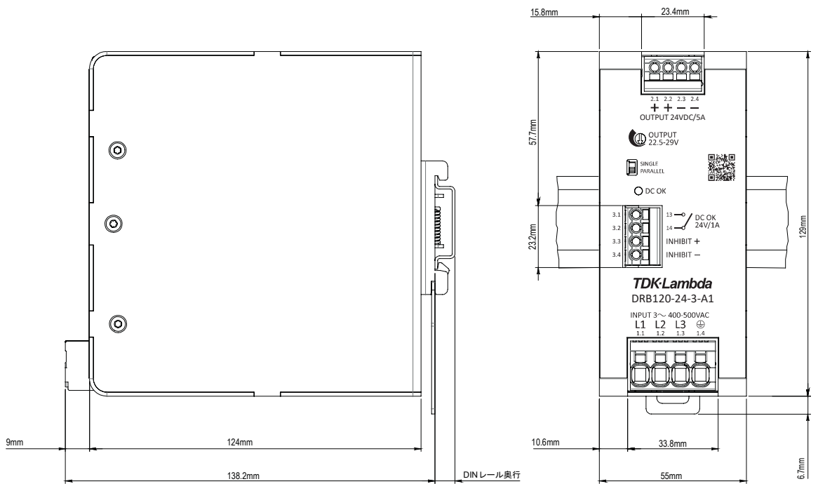
図.22: DRB120-24-3-A1の寸法図
