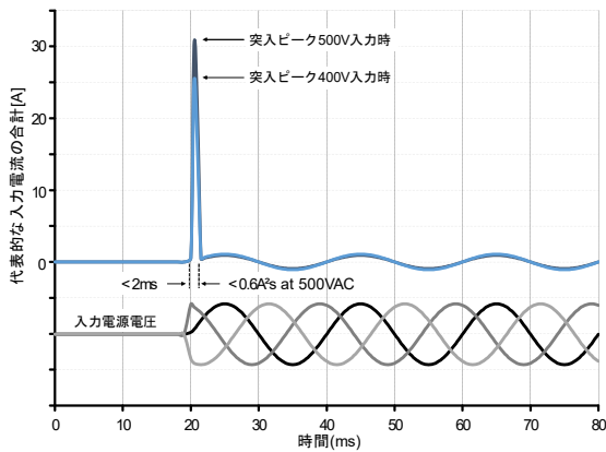
図.5: AC入力投入時の突入電流とエネルギー
