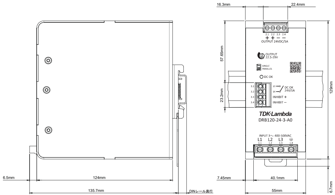
図.21: DRB120-24-3-A0の寸法図
