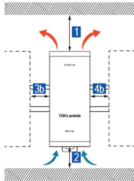
図.24: 受動部品との設置間隔
