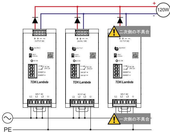
図.32: 冗長性が制限された120Wアプリケーションの例
