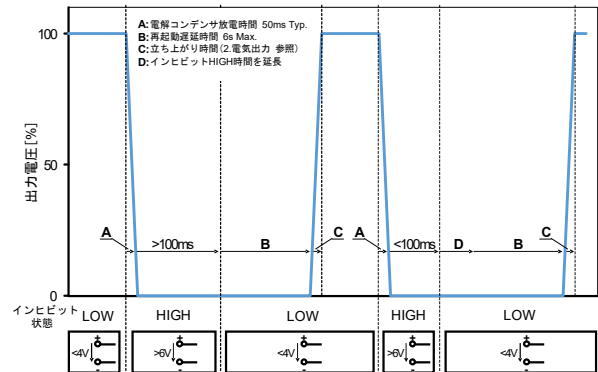
図.26: インヒビット状態に対する出力電圧制御
