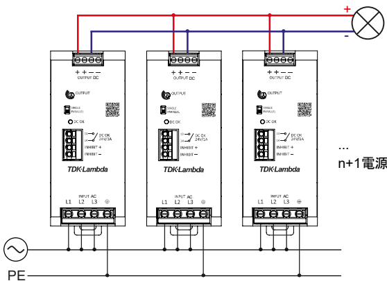
図.30: n+1電源を並列接続するための接続方式
