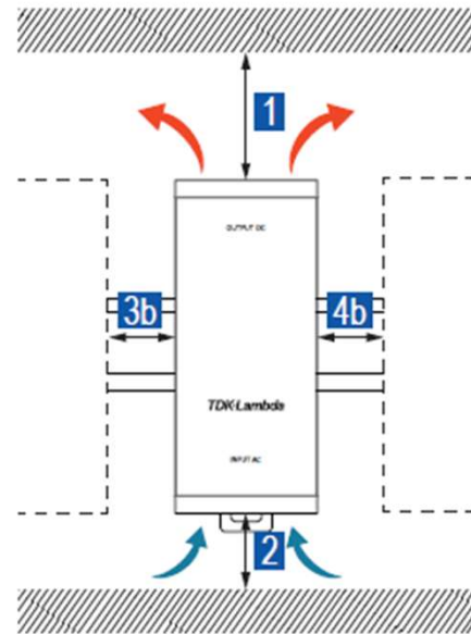
図.24: 受動部品との設置間隔
