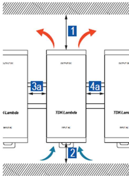
図.23: 熱源との設置間隔
