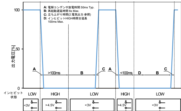
図.26: インヒビット状態に対する出力電圧制御
