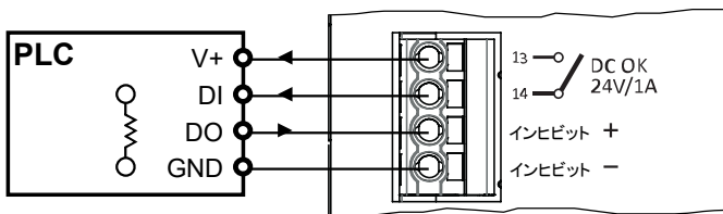
図.27: DC OKおよびインヒビット接点の一般的な接続図
