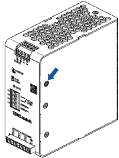
図.29: GDTの接続ねじの位置
