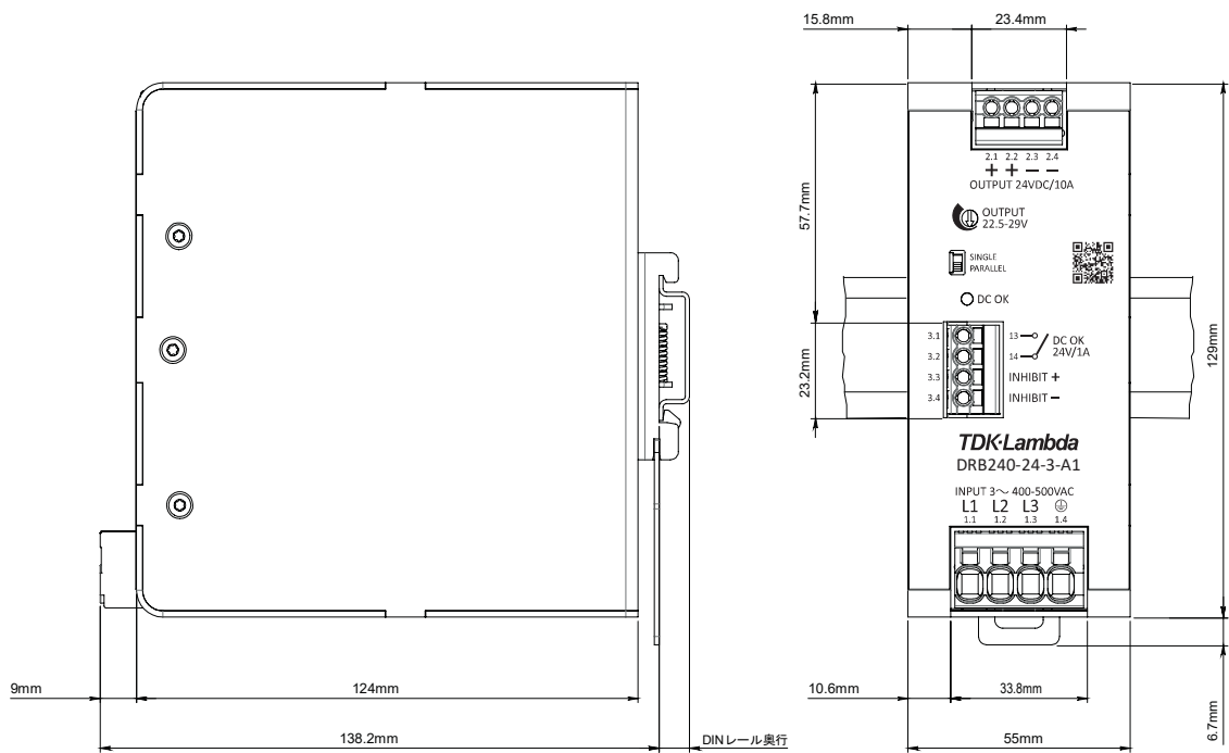
図.22: DRB240-24-3-A1の寸法図
