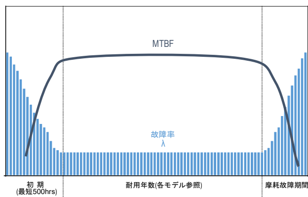
図.20: 製品ライフサイクル中の故障率とMTBF値を視覚化した一般的な図
