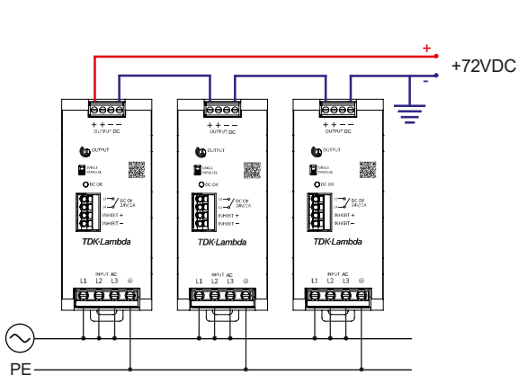
図.34: 正電圧レベルでの直列動作の接続方式
