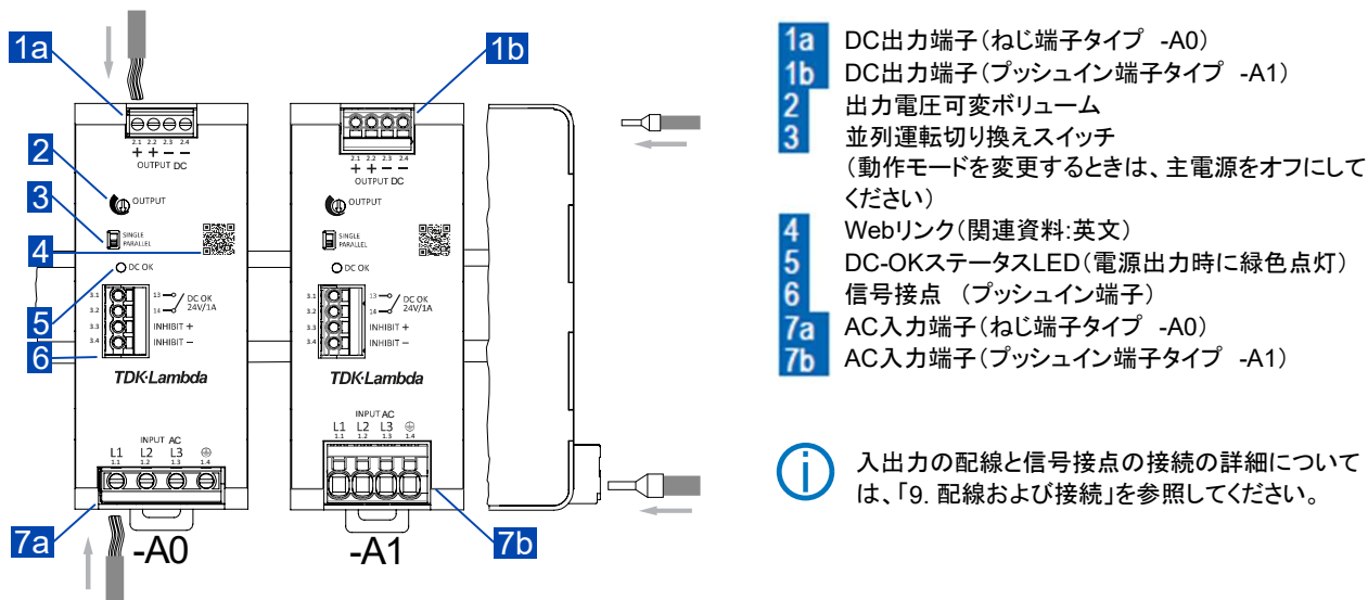
図.1: 端子説明
