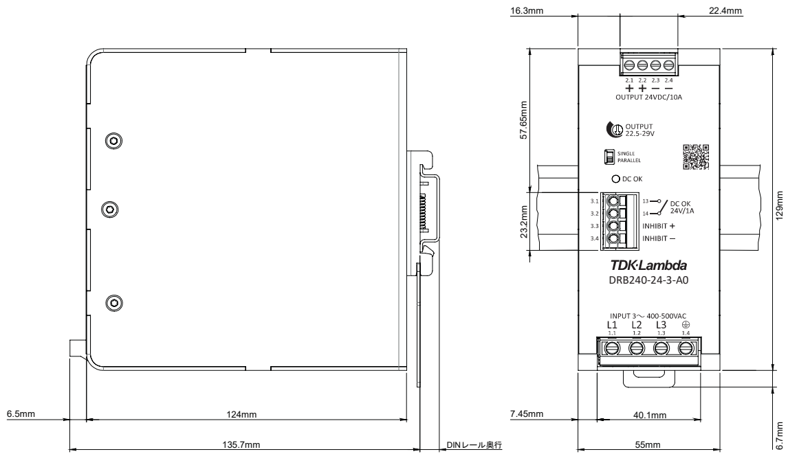
図.21: DRB240-24-3-A0の寸法図
