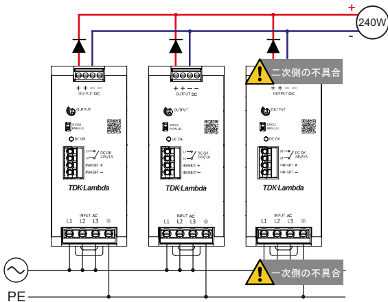
図.32: 冗長性が制限された240Wアプリケーションの例
