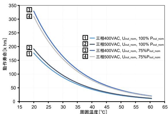
図.19: 電解コンデンサ期待寿命
