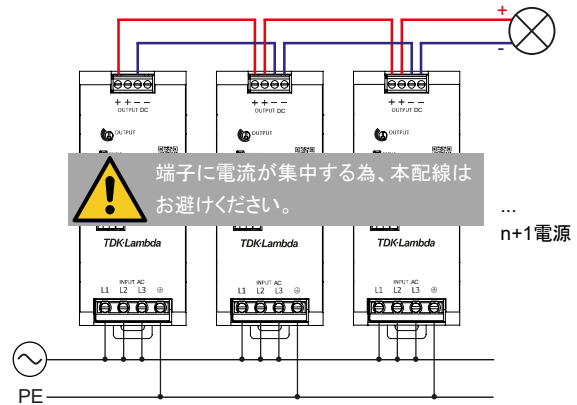
図.31: 誤った並列配線の例
