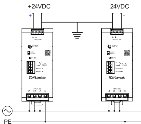
図.36: センタータップによる直列運転の接続方式
