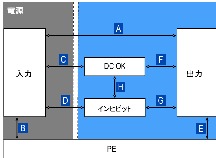
図.28: 絶縁経路の概略図
