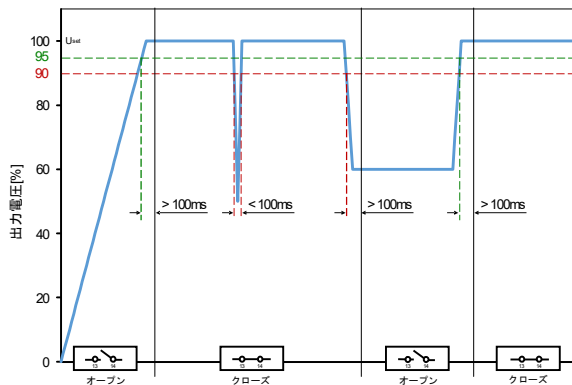
図.25: 出力電圧変動に対するDC-OKリレー特性
