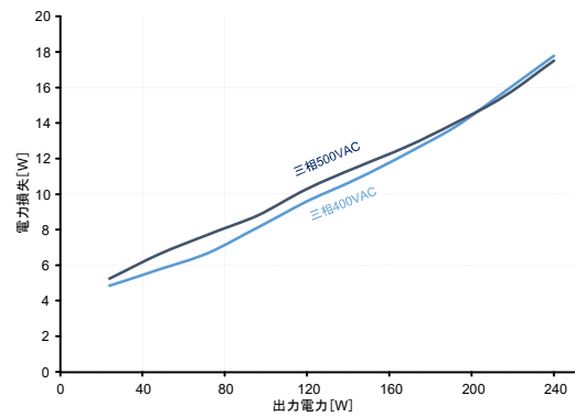
図.8: 出力電力 vs 電力損失
