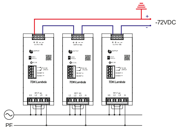
図.35: 負電圧レベルでの直列動作の接続方式
