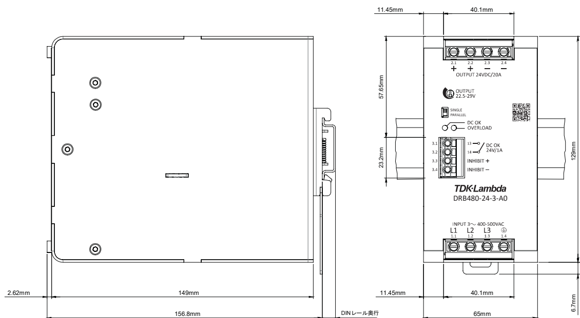
図.22: DRB480-24-3-A0の寸法図
