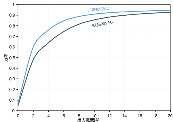
図.9: 出力電流 vs 力率
