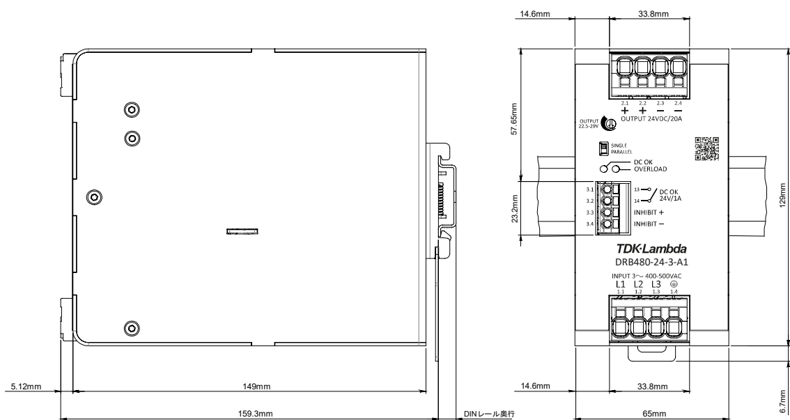
図.23: DRB480-24-3-A1の寸法図
