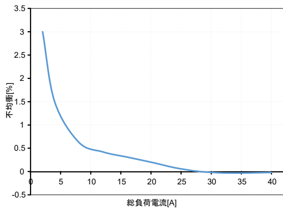
図.34: 並列動作における2台の電源装置の負荷分散動作例
