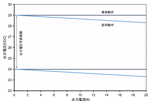
図.4: 並列動作時における出力電圧低下特性
