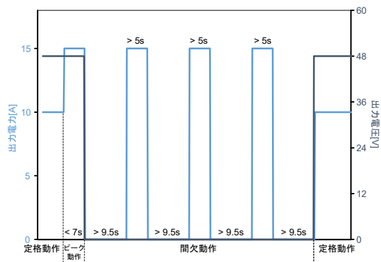
図.3: 出力電流条件における各動作モード
