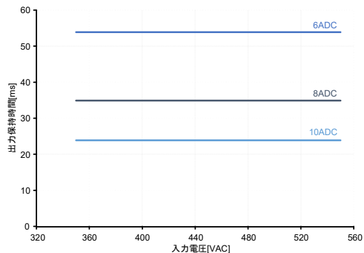
図.2: 入力電圧 vs 出力保持時間 (出力電流別)
