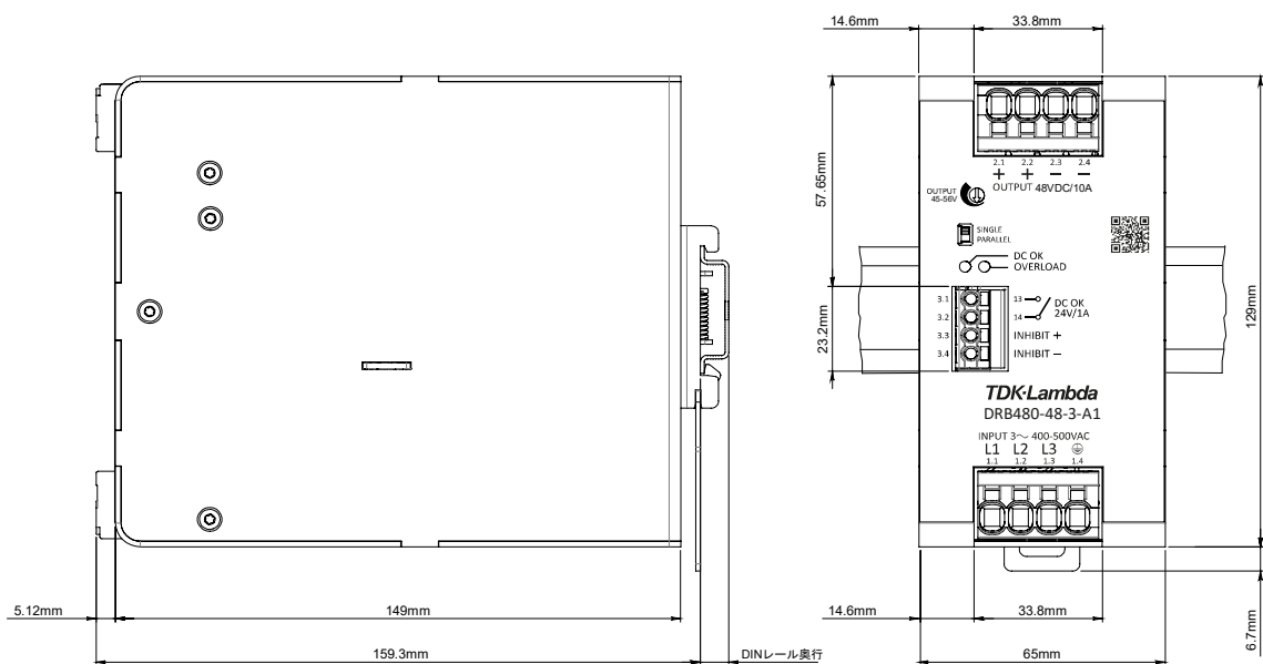
図.23: DRB480-48-3-A1の寸法図
