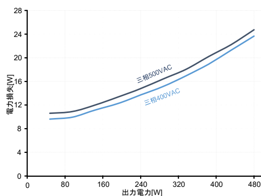
図.8: 出力電力 vs 電力損失
