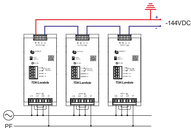
図.36: 負電圧レベルでの直列動作の接続方式
