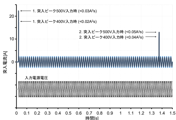
図.5: AC入力投入時の突入電流とエネルギー
