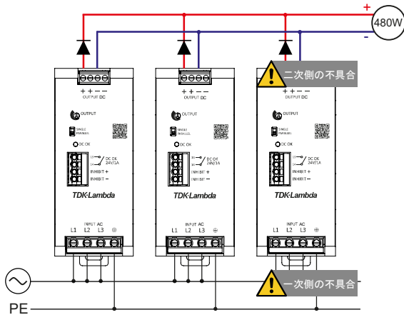
図.33: 冗長性が制限された480Wアプリケーションの例
