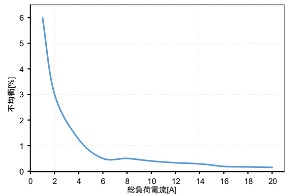
図.34: 並列動作における2台の電源装置の負荷分散動作例
