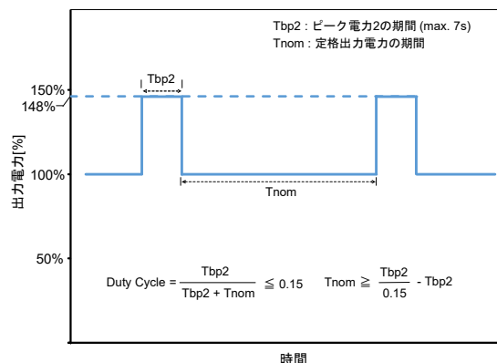
図.11: 標準取付位置でのピーク電力2のサイクル図
