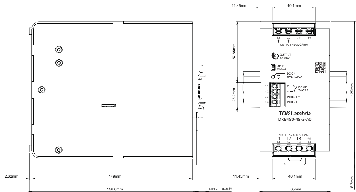
図.22: DRB480-48-3-A0の寸法図
