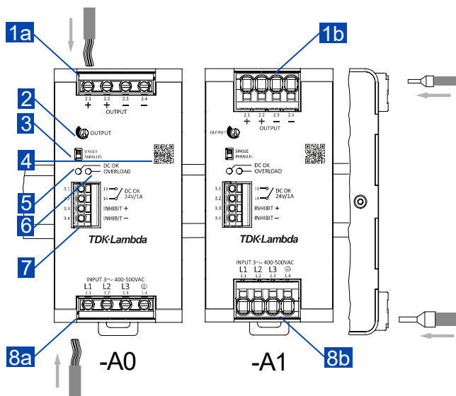
図.1: 端子説明
