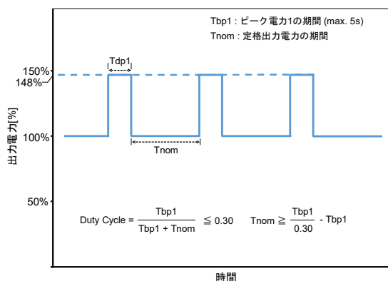
図.10: 標準取付位置でのピーク電力1のサイクル図
