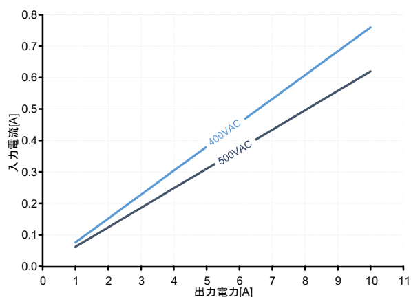
図.6: 出力電流 vs 入力電流 (線電流)
