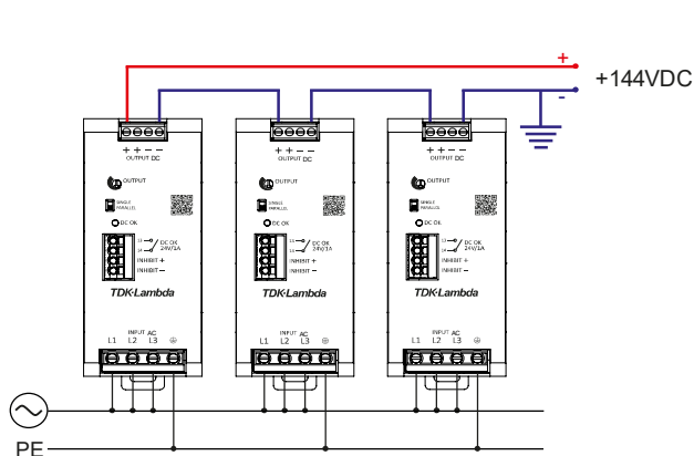
図.35: 正電圧レベルでの直列動作の接続方式
