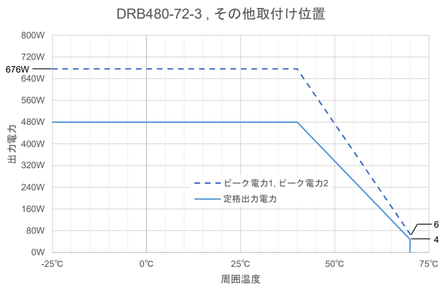
図.13: 取付け位置 (図.15 - 図.19) での電力ディレーティング
