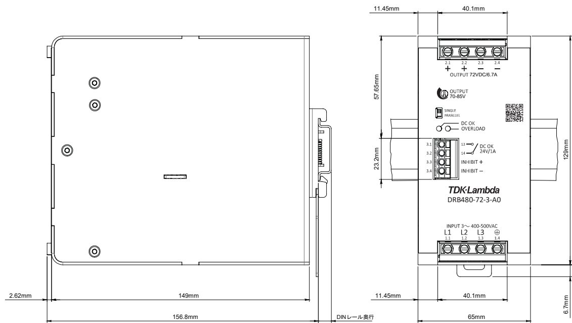
図.22: DRB480-72-3-A0の寸法図
