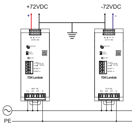
図.37: センタータップによる直列運転の接続方式
