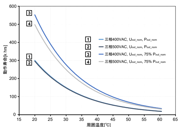
図.20: 電解コンデンサ期待寿命
