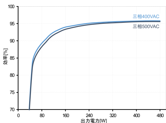
図.7: 出力電力 vs 効率
