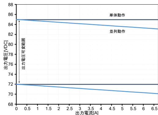
図.4: 並列動作時における出力電圧低下特性
