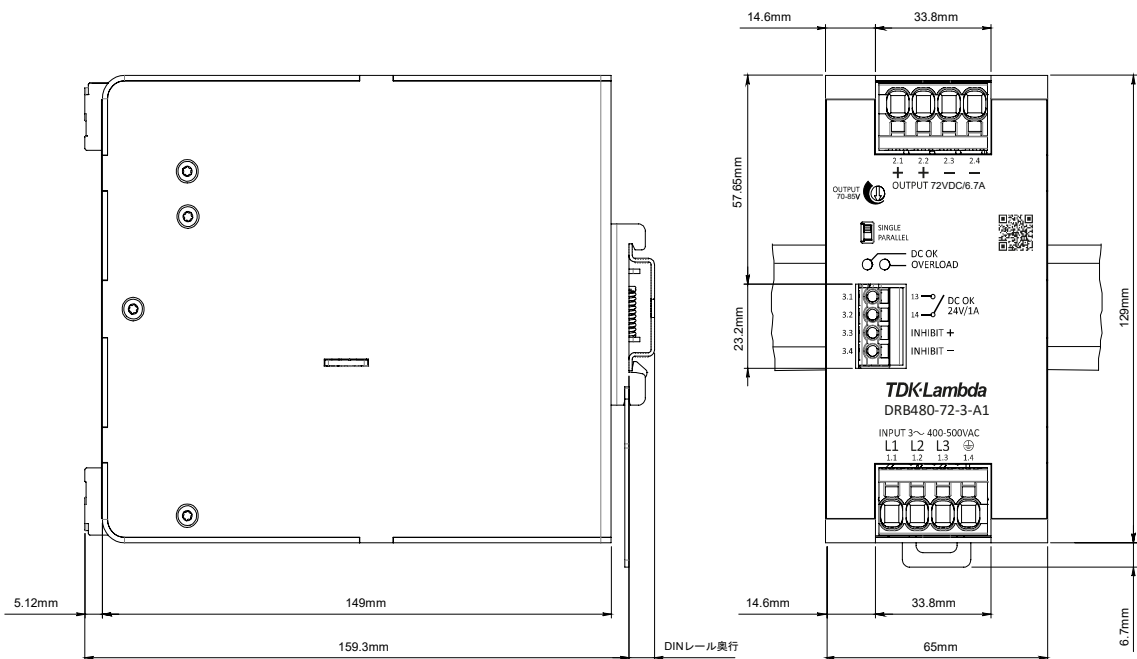
図.23: DRB480-72-3-A1の寸法図
