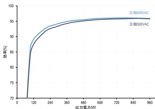
図.7: 出力電力 vs 効率
