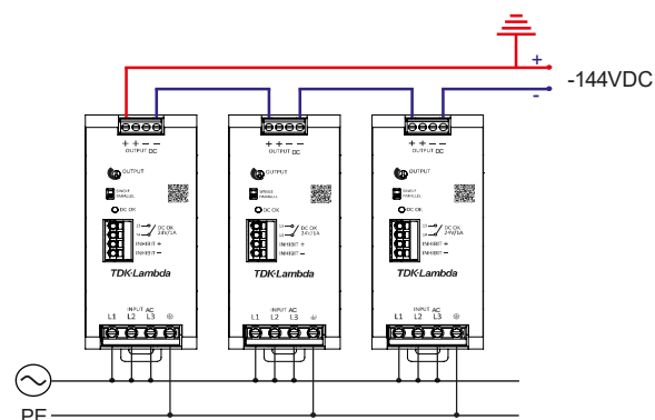
図.36: 負電圧レベルでの直列動作の接続方式
