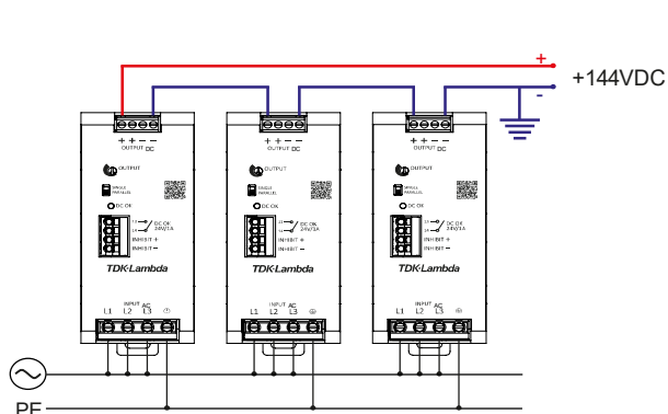
図.35: 正電圧レベルでの直列動作の接続方式
