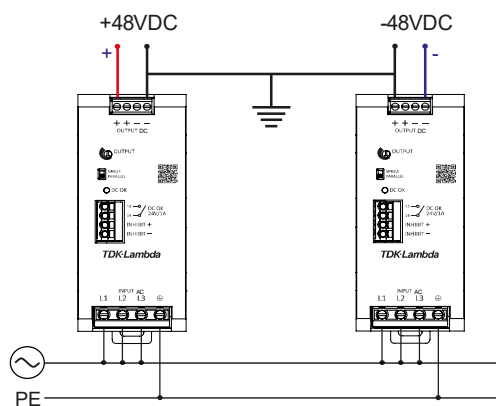
図.37: センタータップによる直列運転の接続方式
