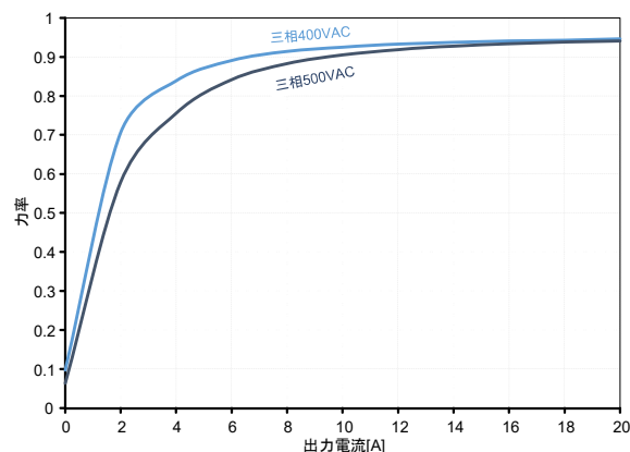
図.9: 出力電流 vs 力率
