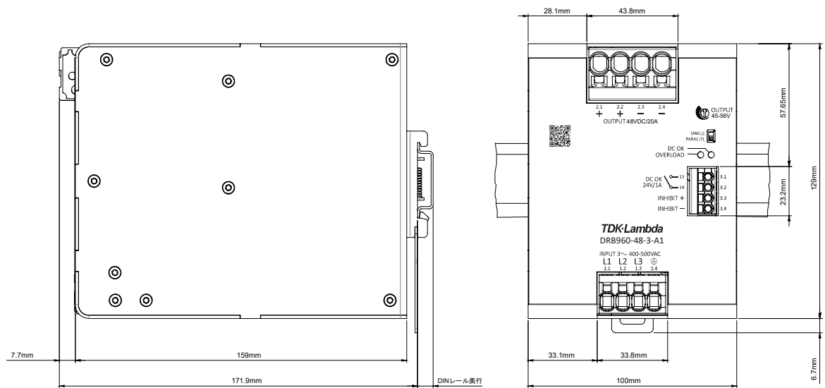
図.23: DRB960-48-3-A1の寸法図
