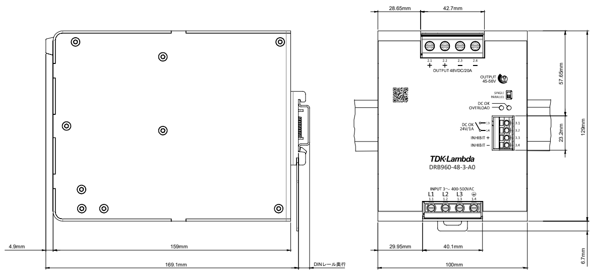
図.22: DRB960-48-3-A0の寸法図
