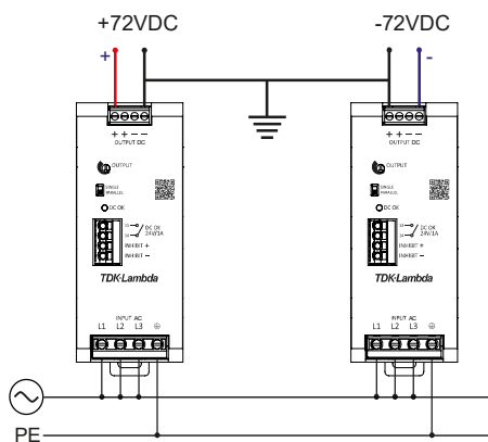
図.37: センタータップによる直列運転の接続方式
