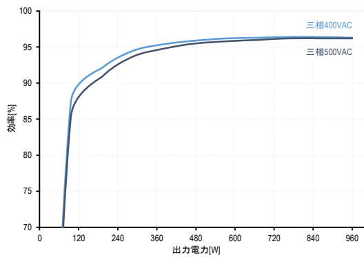
図.7: 出力電力 vs 効率
