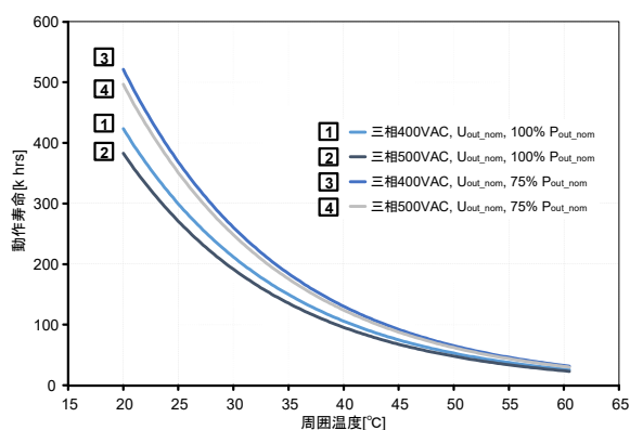
図.20: 電解コンデンサ期待寿命
