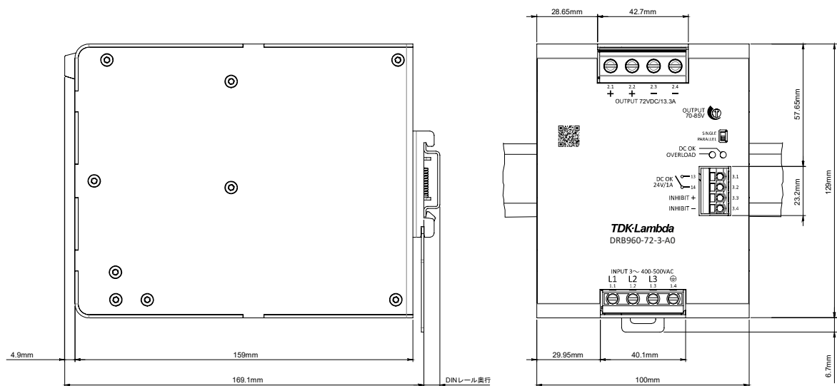
図.22: DRB960-72-3-A0の寸法図
