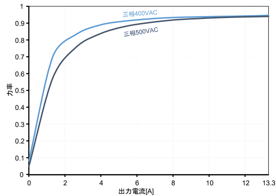
図.9: 出力電流 vs 力率
