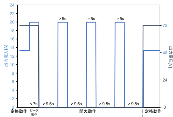
図.3: 出力電流条件における各動作モード
