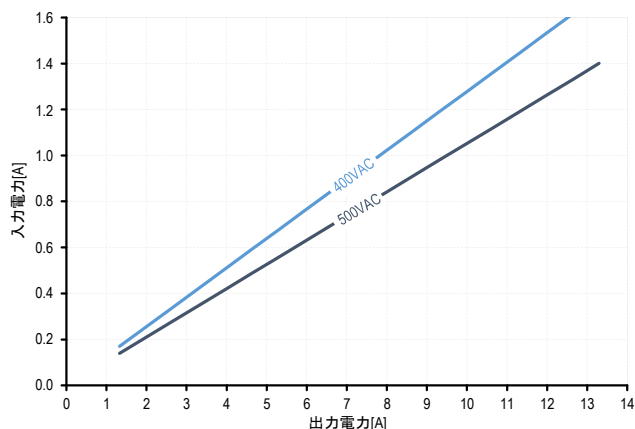
図.6: 出力電流 vs 入力電流 (線電流)
