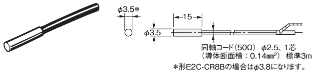
形E2C-X1A
