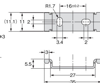
取付金具
