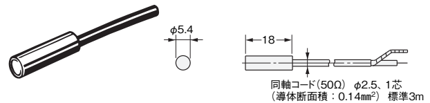
形E2C-X2A
