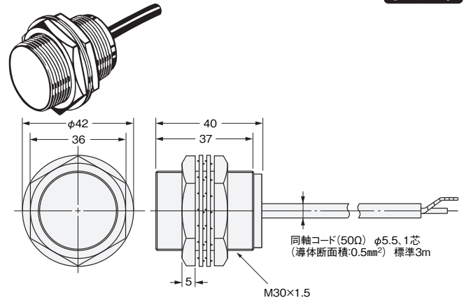
形E2C-X10A
