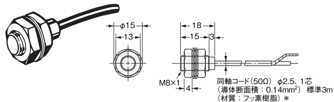
形E2C-X5A
