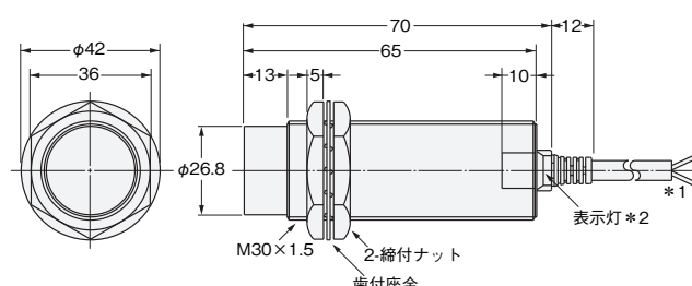
形E2E2-X20MD□/形E2E2-X18MC□/形E2E2-X18MY□
