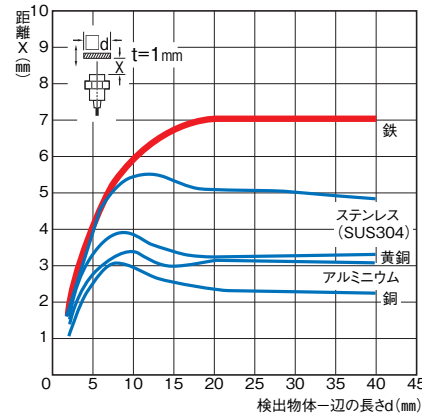
形E2EQ-X7D1(-M1(T)GJ)
