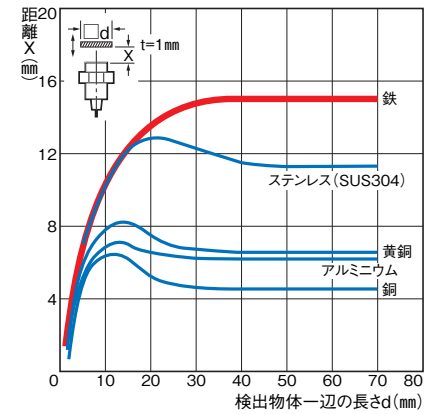
形E2EQ-X10D1(-M1(T)GJ)
