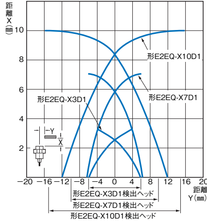
形E2EQ-X□D□(-M1(T)GJ)
