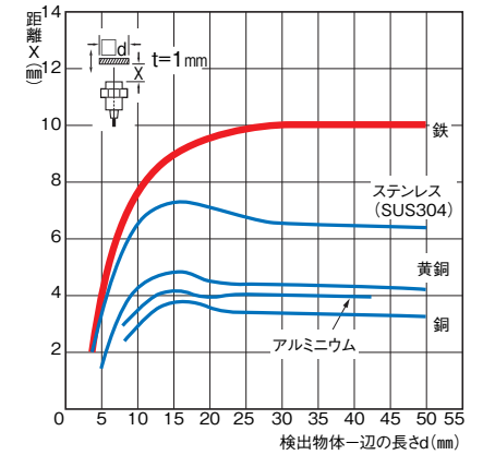
形E2EQ-X10D1(-M1(T)GJ)
