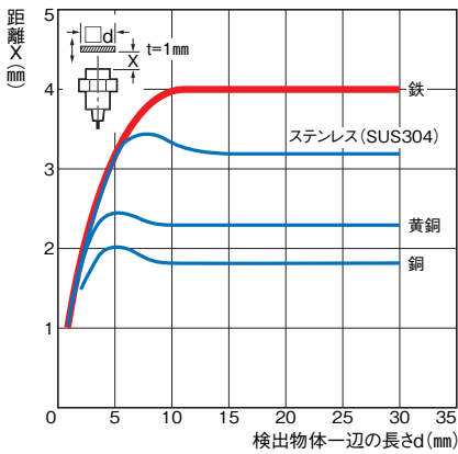
形E2EQ-X3D1(-M1(T)GJ)
