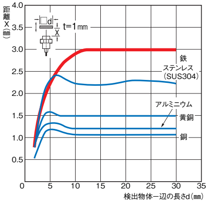
形E2EQ-X3D1(-M1(T)GJ)
