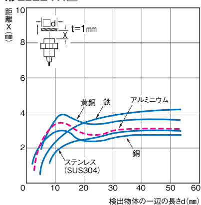
形E2EZ-X4□
