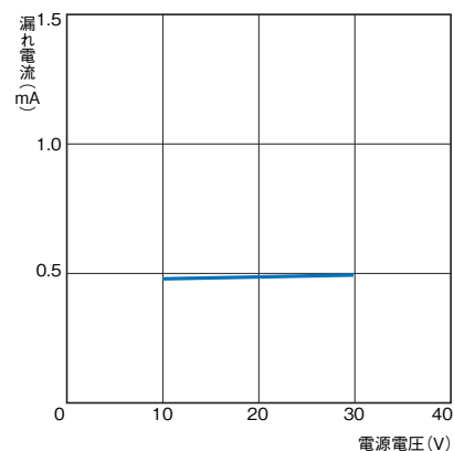
形E2EZ-X□D□-N
