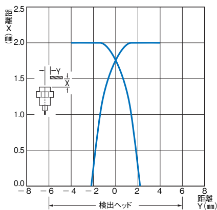
形E2EZ-X2□
