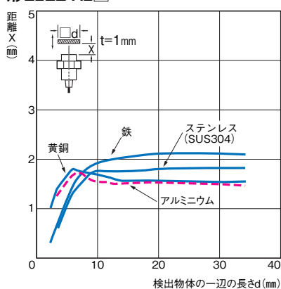
形E2EZ-X2□
