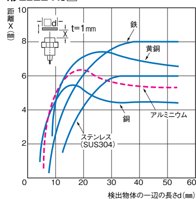
形E2EZ-X8□
