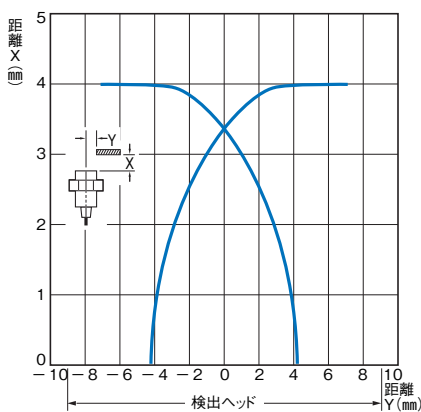
形E2EZ-X4□
